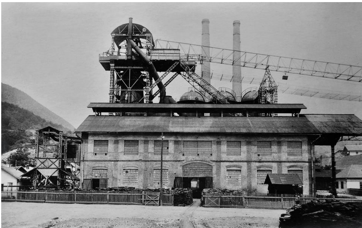
Druhá lanovka celkom vľavo dopravujúcou vysokopecnú trosku na skládku a tretia lanovka na pevnej nosnej konštrukcii medzi rudným dvorom a kychtou vysokej pece.
