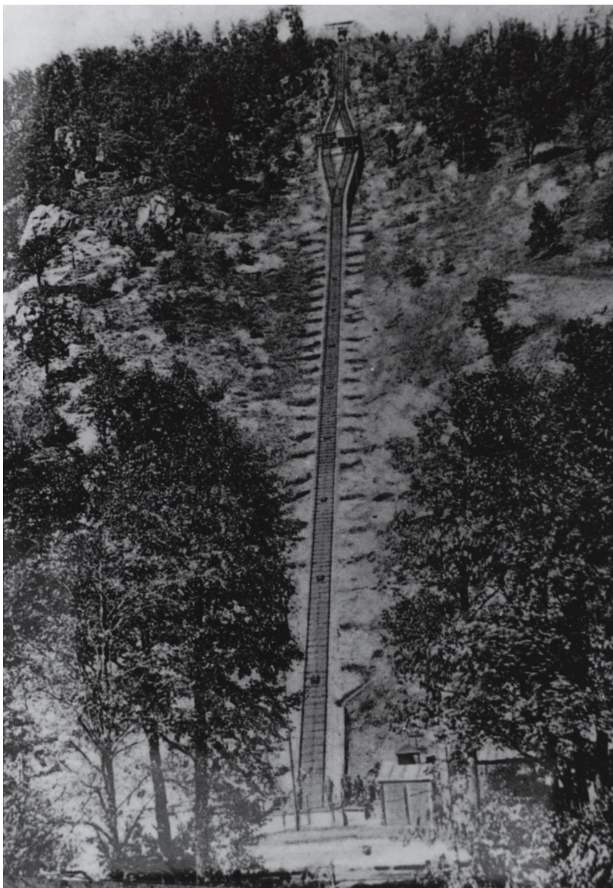
Pohľad na dvojkoľaj pozemnej lanovky Šiklov s vozíkmi stretávajúcimi sa vo výhybni.
