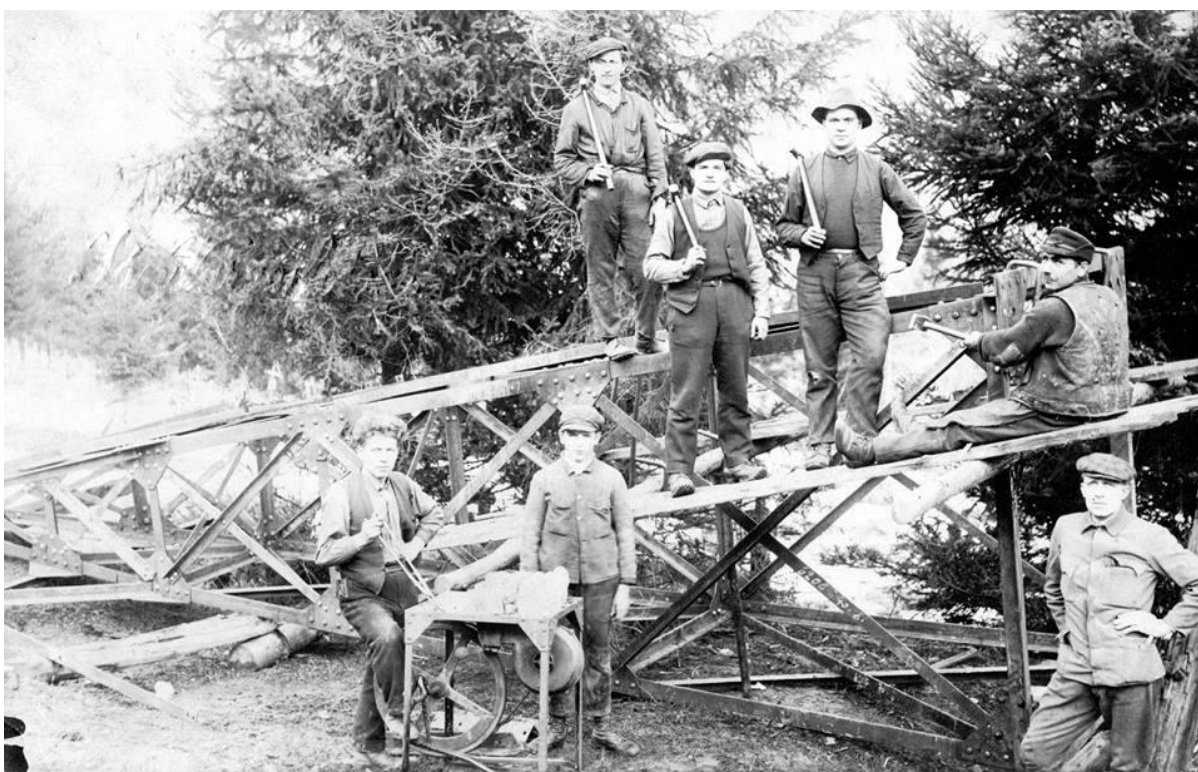
Výmena pôvodných drevených stožiarov za oceľové. Konštrukcia sa zostavovala na mieste nitovaním za pomoci prenosnej vyhne s nožným dýchadlom.
