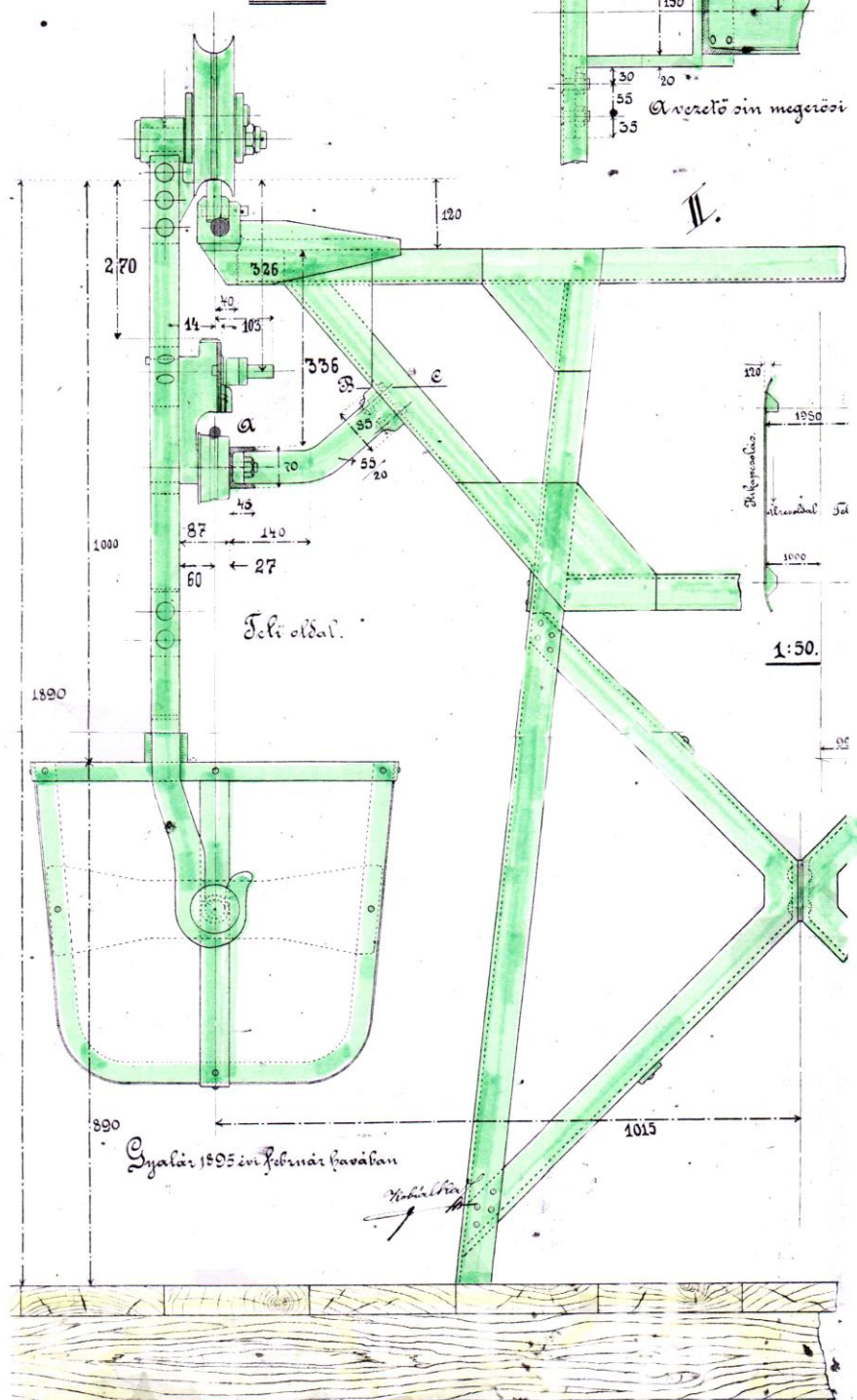
Detail lanovkového výsypného vozíka s pojazdom po nosnom lane (hore). Pod ním aretačný mechanizmus ťažného lana s menším priemerom.
