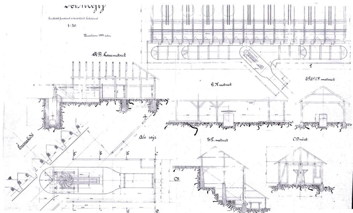
Plán nakladacej stanice pred štôľňou František Jozef so zásobníkom rudy so sýpmi a nakladacou slučkou lanovky a napínacou kladkou (lanáčom) ťažného lana.
