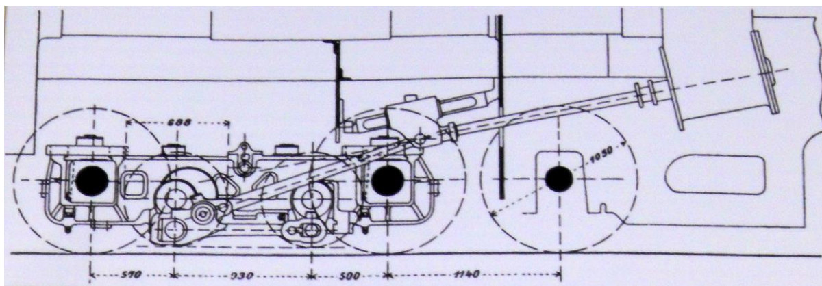
Usporiadanie ozubnicového pojazdu parného rušňa.
