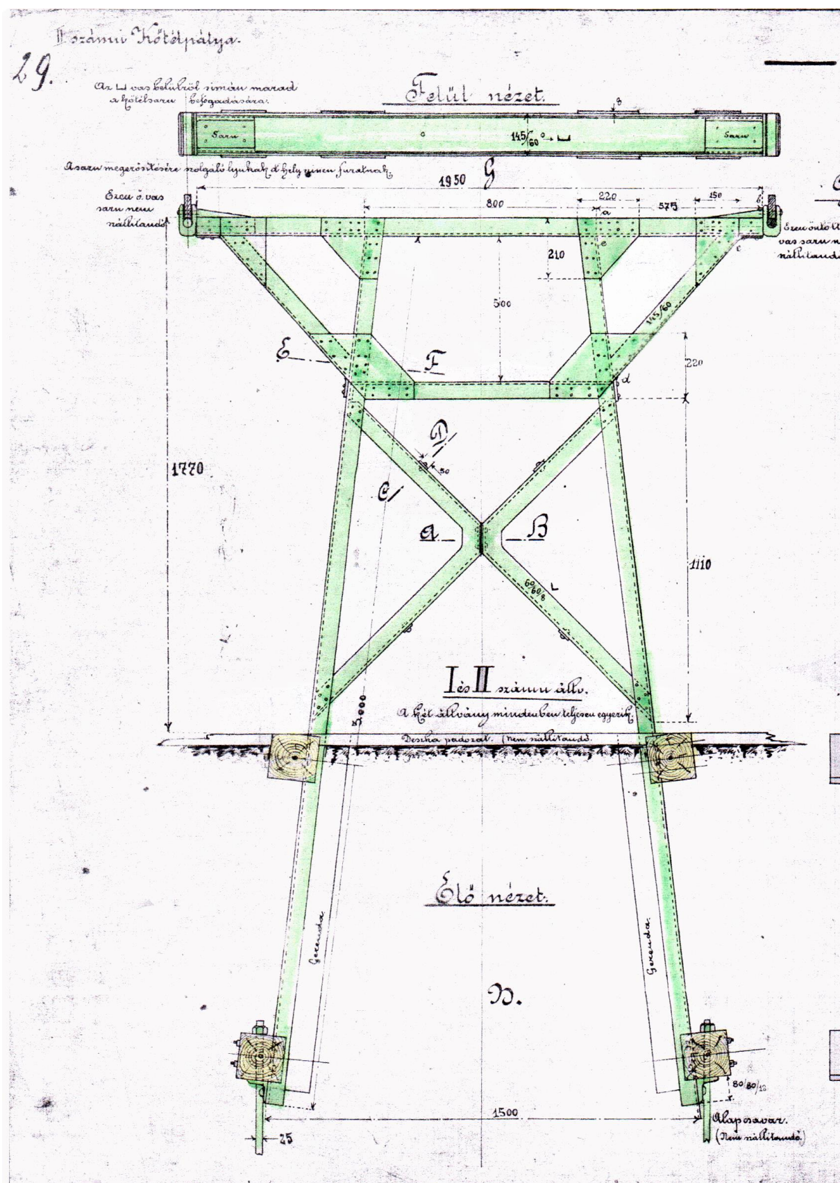
Konstrukcia ocel'ového nosníka lán lanovej dráhy. Všetky vymenili za pôvodné dubové v medzivojnovom období.
