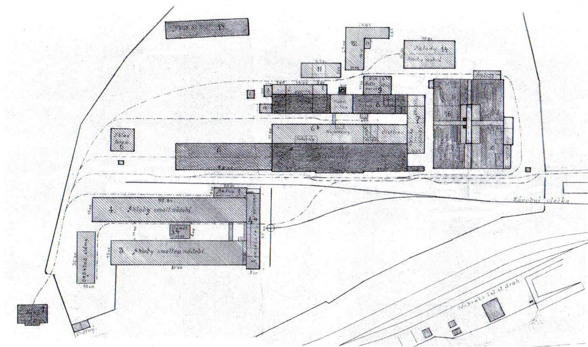
Časť železničnej site v zlievarni Hronec: čiarkovane fabrický úzkokolejka, plná čiara normálnorozchodná trať. Vpravo dole železničná stanica, vľavo dole vážnica a hlavná brána.
