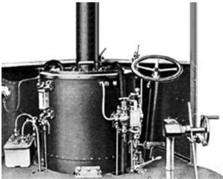
Interiér kabíny automobilu Škoda-Sentinel s vertikálnym kotlom uprostred s komínom.
