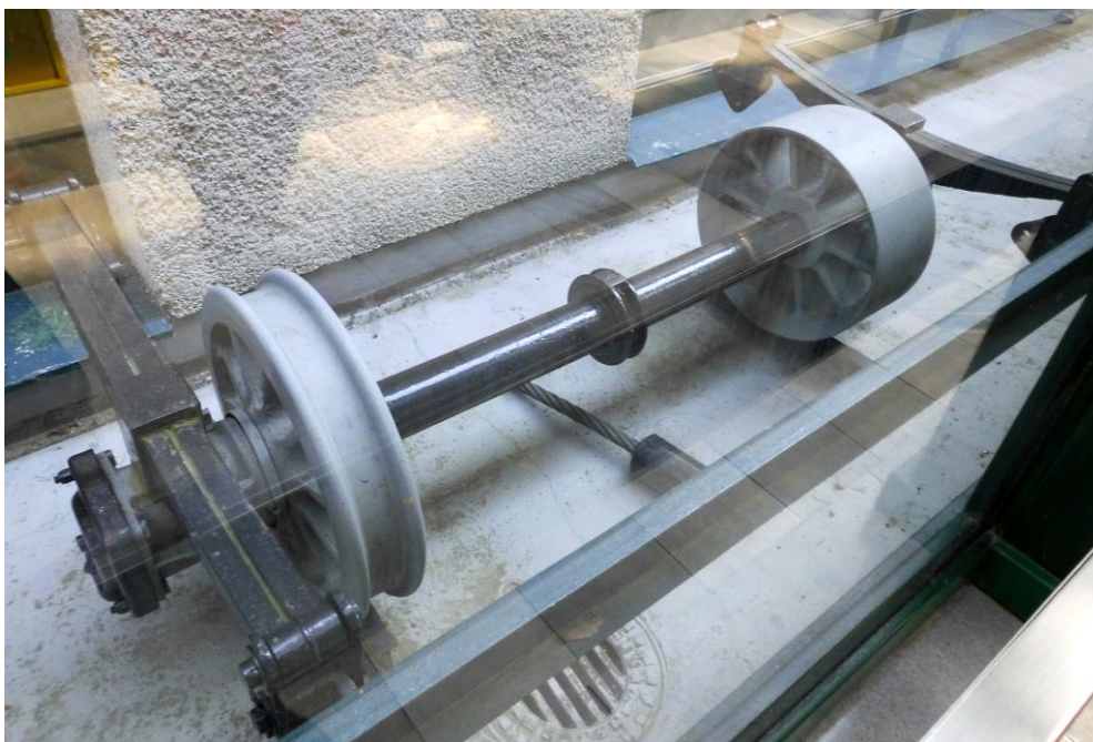
Ilustračné foto na súkolie vozíka pozemnej lanovky s vodiacim kolesom s okolesníkom po oboch stranách pre vonkajšiu koľaj výchybne a vnútorné koleso bez okolesníka na prechod z jednej koľaje na druhú bez potreby pohyblivej časti výmeny.
