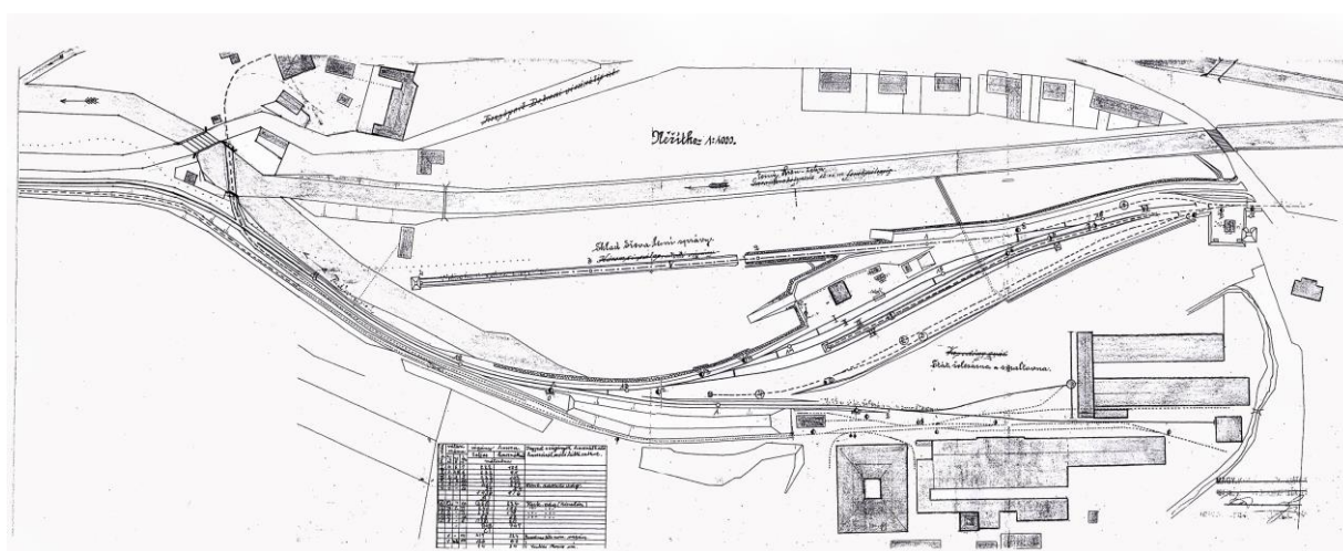
Plán železničnej stanice v Hronci s fabrickou vlečkou a vlečkou štátnych lesov. Dole vpravo zlievareň a smaltovňa, hore vľavo lisovňa plechového riadu s podnikovou železničkou (čiarkovane). Uprostred pôvodný plavebný kanál rozšírený na nové koryto Čierneho Hrona. Zvyšok starého koryta ešte poznať vľavo dole. Ostatnú časť zasypali pri stavbe koľajiska.
