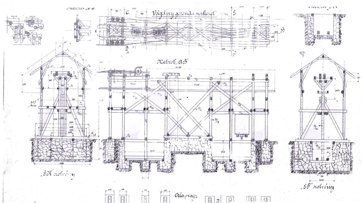
Drevená napínacia stanica, kde sa napínali nosné laná lanovej dráhy.
