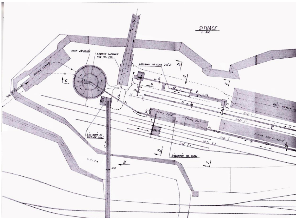
Plán hutného dvora v Tisovci so železničnou vlečkou (plné čiary) a lanovou dráhou (čiarkovane) s prijímacou stanicou, kruhovým sklodom (bunkrom) triedenej rudy.
