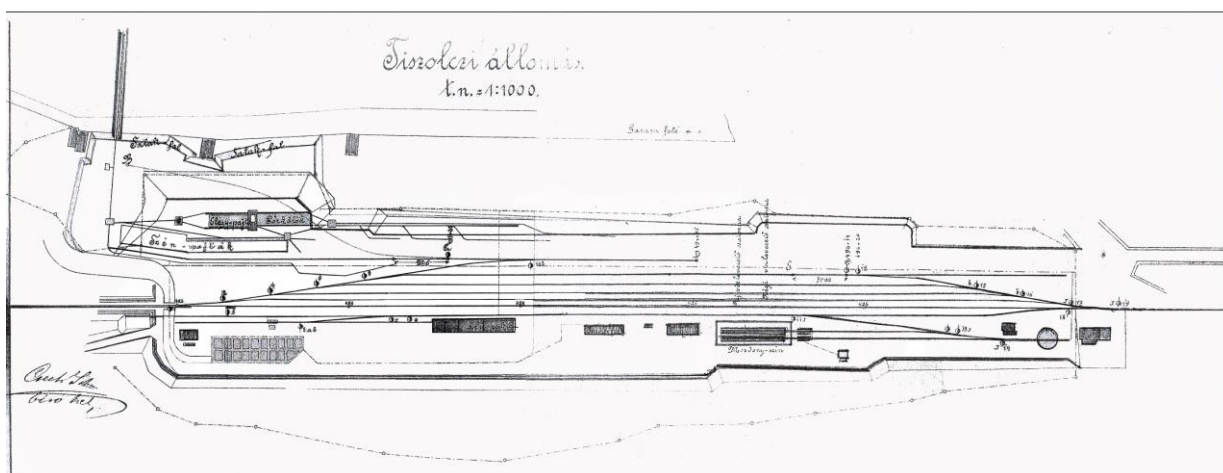
Železničná stanica Tisovec v r. 1897 s traťou vľavo smer Jesenské a vpravo s točňou smer Brezno. Hore vľavo vlečka pre rudný dvor vysokej pece ešte bez prijímacej stanice lanovky.
