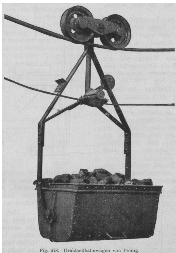
Vozík (huntík) nákladnej lanovky s pojazdovým dvojkolím a aretačným mechanizmom.
