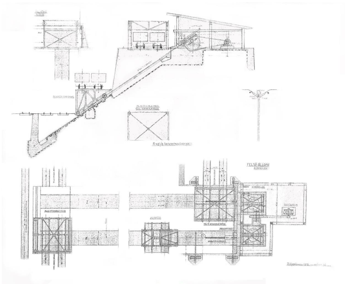
Plán podbrezovskej pozemnej lanovky z r. 1912 ešte s dvojicou súbežných koľají bez výhibne.
