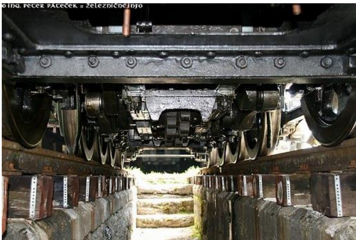
Pohľad pod lokomotivu na súkolia adhézneho pojazdu a v strede ozubeného súkolia.
