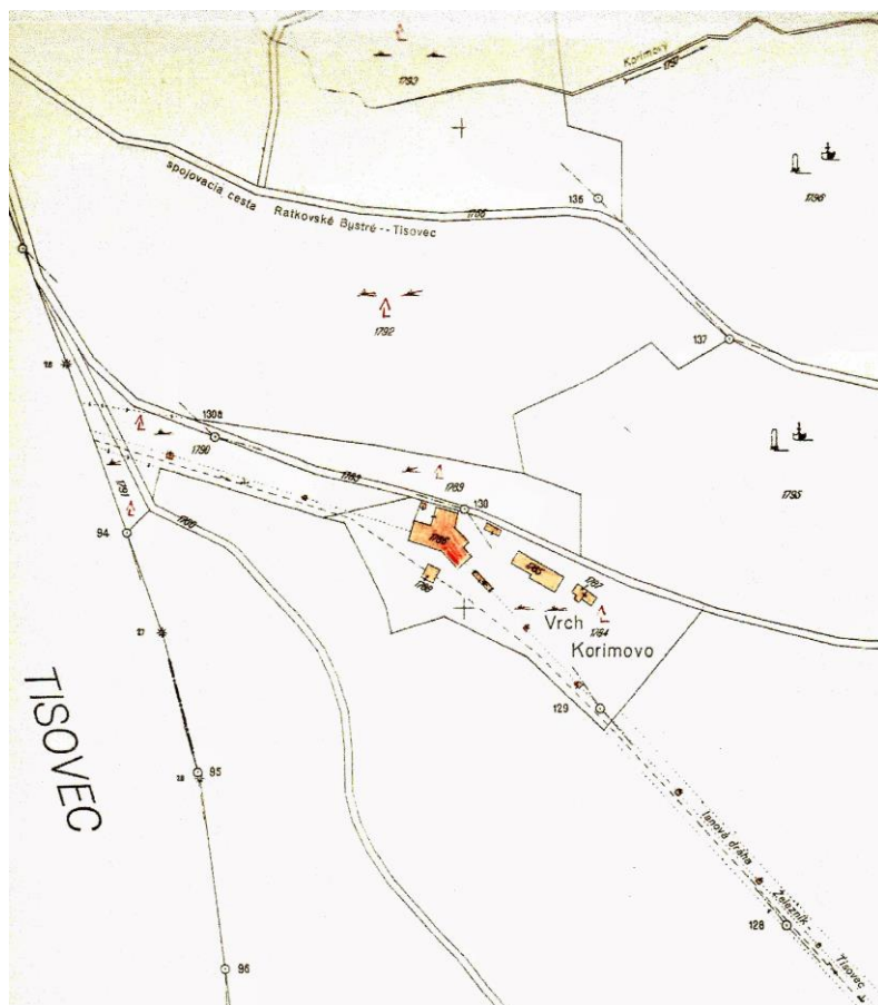
Poháňacia stanica lanovky Ratkovské Bystré so zalomením dráhy lanovky medzi nakladacou stanicou v Sirku a druhej pohonnej stanice lanovky Korimovo.
