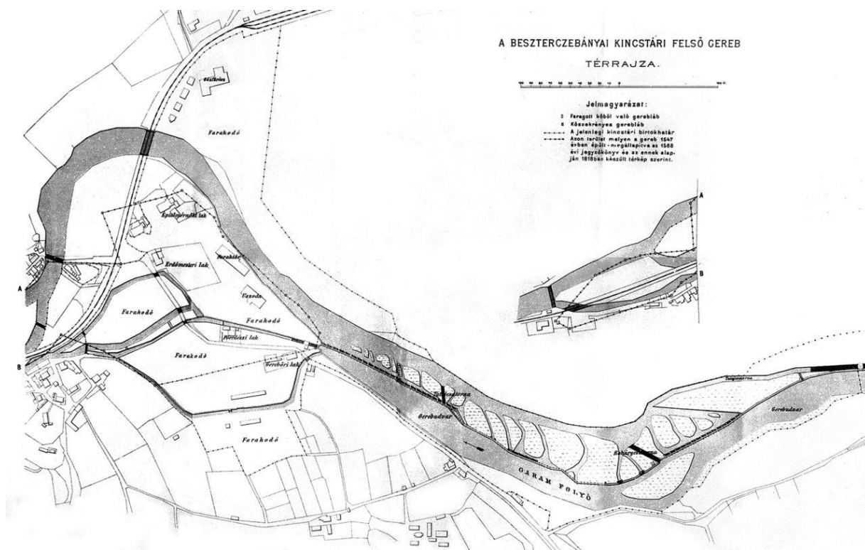
Plán banskobystričských horných hrablí: vľavo hore železničná stanica, vpravo pltný priepust.
