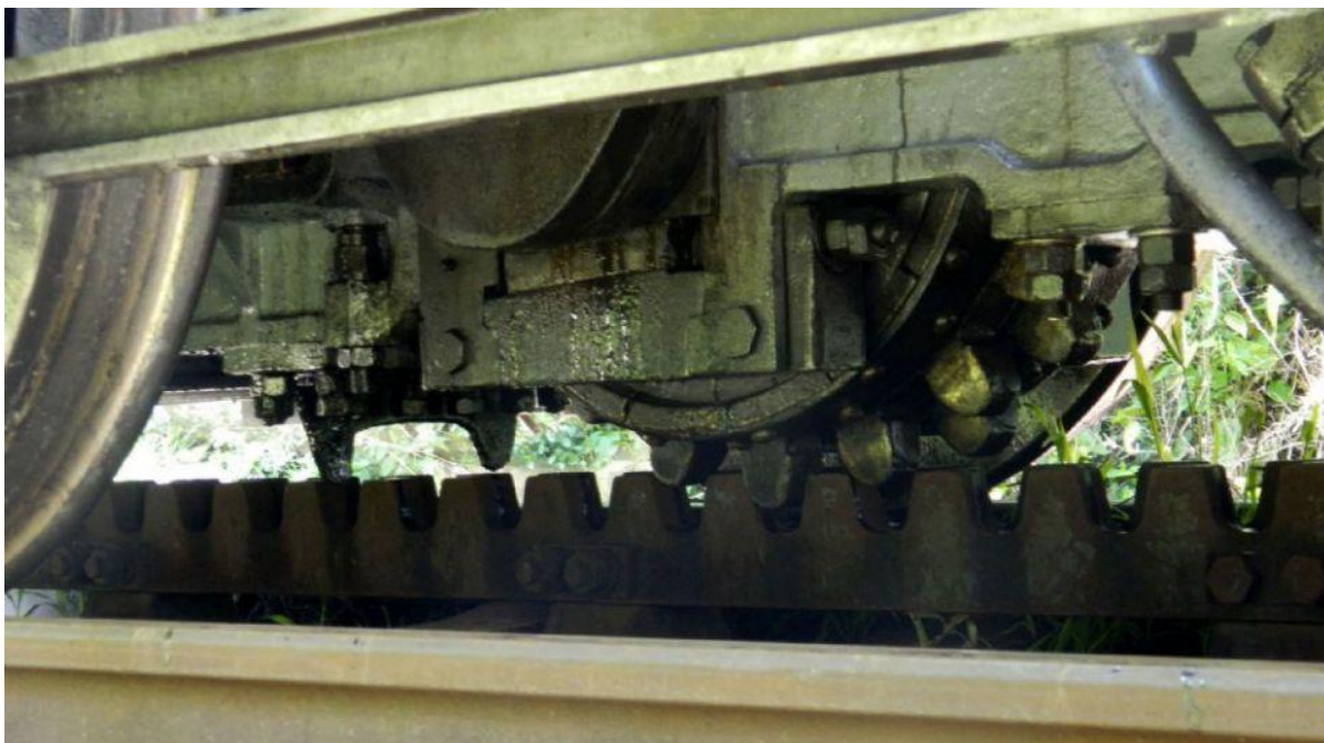
Abtov systém trakcie ozubeným dvojkoľím zaberajúcim do dvojitého hrebeňa osadeného v strede koľají.
