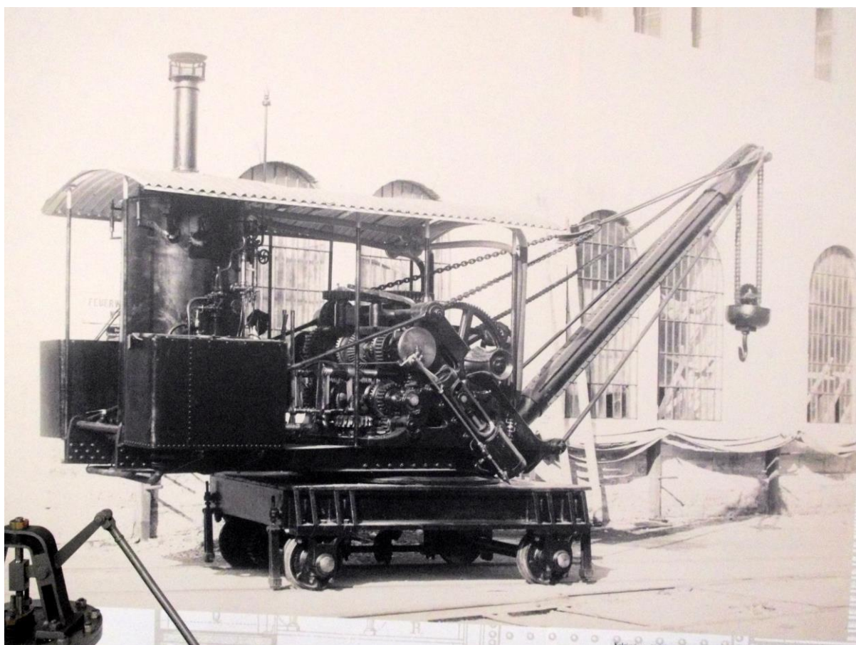
Továrenská fotografia parného koľajového žeriavu aký zakúpila aj podbrezovská železiareň.
