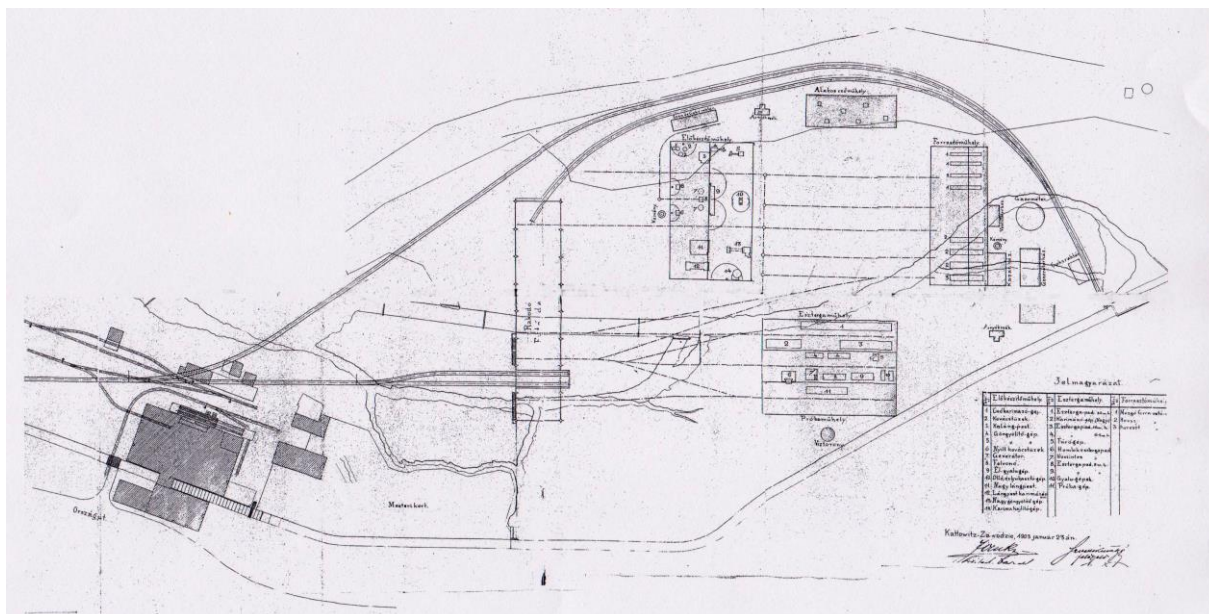
Železničná sieť v Henriho závode v Piesku: prerušovane fabrická železnička, plná dvojitá čiara normálnerozchodná trať podnikovej vlečky, vľavo dole stará valcovňa na vodný náhon, od stredu doprava nová fabrika Henriho závod, celkom vpravo kyslíkareň s plynojemom.
