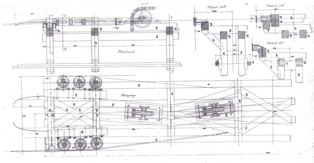
Detail umiestnenia kladiek napínacej stanice v bočnom pohľade a pôdoryse. Zľava nábehové lyžiny nosného lana a batérie vychýľovacích kladiek. Priamo pokračuje koľajnica na opačný okraj napínacej stanice kde sa nábehovou lyžinou opäť spojila s ďalším lanovým úsekom. Uprostred napínacia kladka nosného lana meníaca jeho vodorovné napínanie 90 stupňovým ohybom do vertikálnej polohy ukončeného napínaním závažím.
