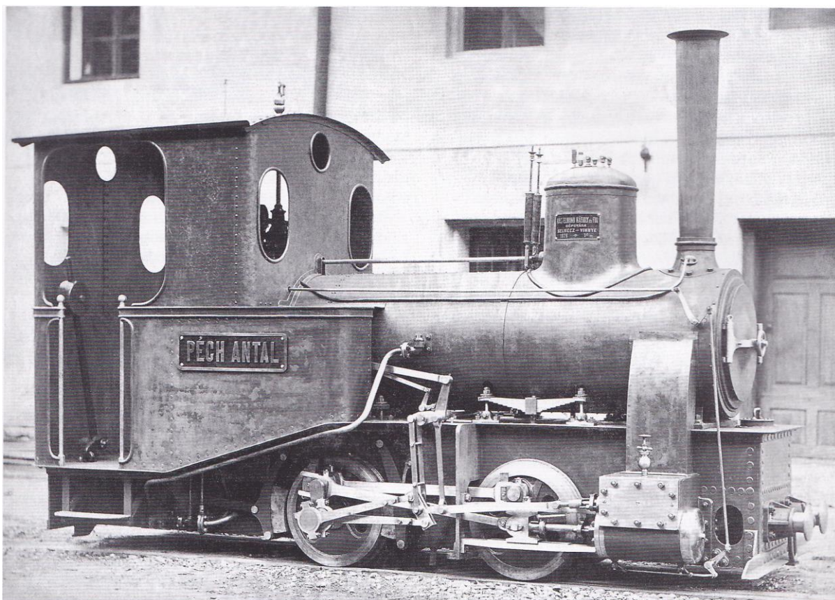
Fabrické foto kachelmanovej lokomotívy vyrobenej pre Hronecký železarský komplex.
