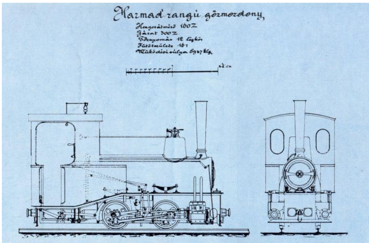
Technický výkres prvej parnej lokomotívy vyrobenej na Slovensku v Kachelmanových železiarňach (zlievárne a strojárne) vo Vyhniach kde vyrábali pre bane banskej komory najmä strojné zariadenia, vodotiažne stroje, vodné turbíny. Tu bol vyrobený aj prvý Wattov ohňový stroj (predchodca parného stroja) pre šachtu v Novej Bani v r. 1722.
