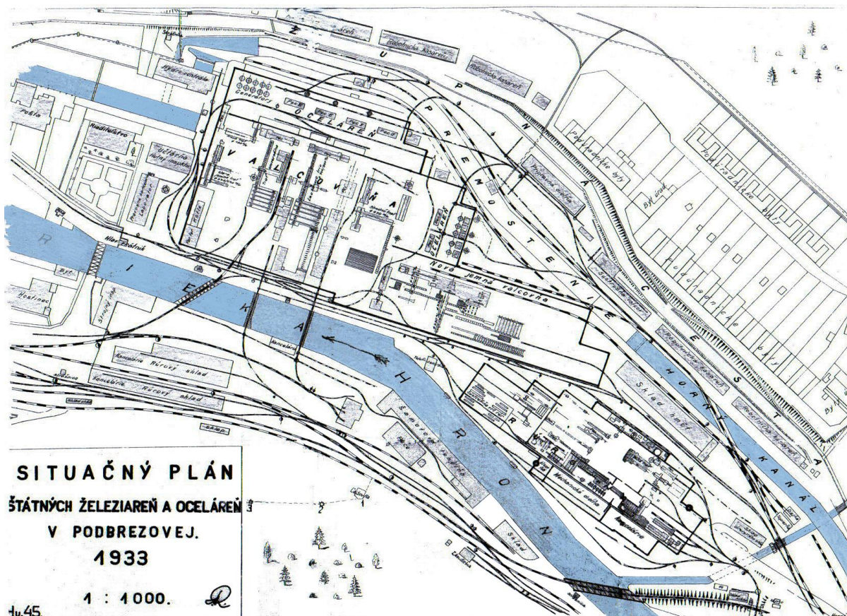
Plán štátnych železiarní v Podbrezovej z r. 1933 s bohato rozvetvenou železničnou sieťou.
