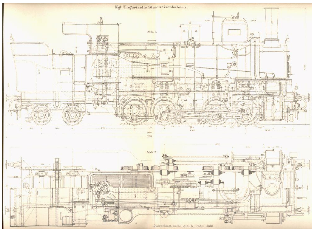
Plán parného rušňa tisovskej ozubnice kategórie TIVb MAV, po r. 1918 radou 403.502 ČSD.
