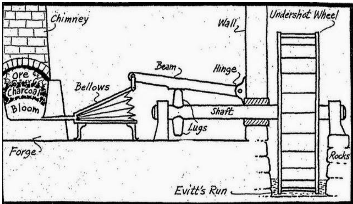
Schématická zostava vyhne, dúchadla a pohonnej jednotky vodným kolesom.
