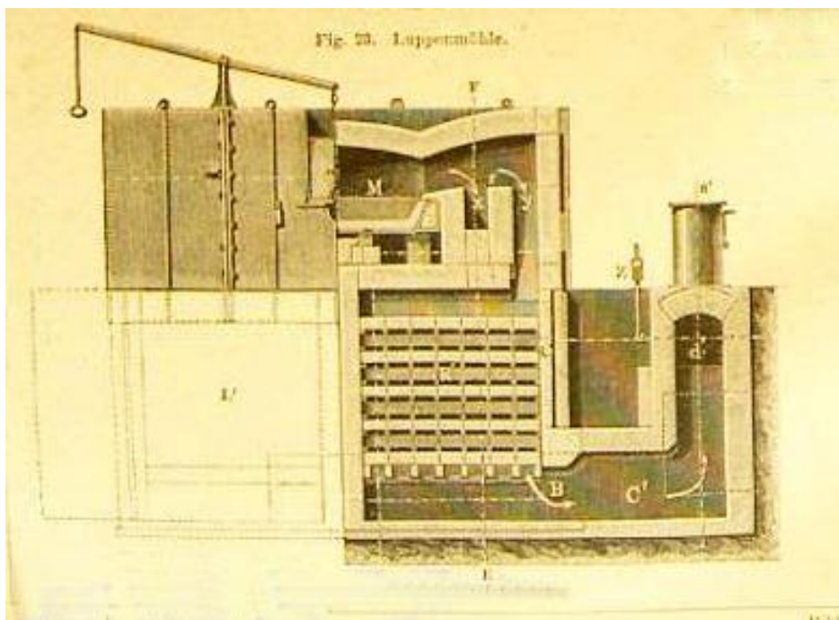
Pudlovacia pec s rekuperátorom odpadného tepla a dymovodom.
