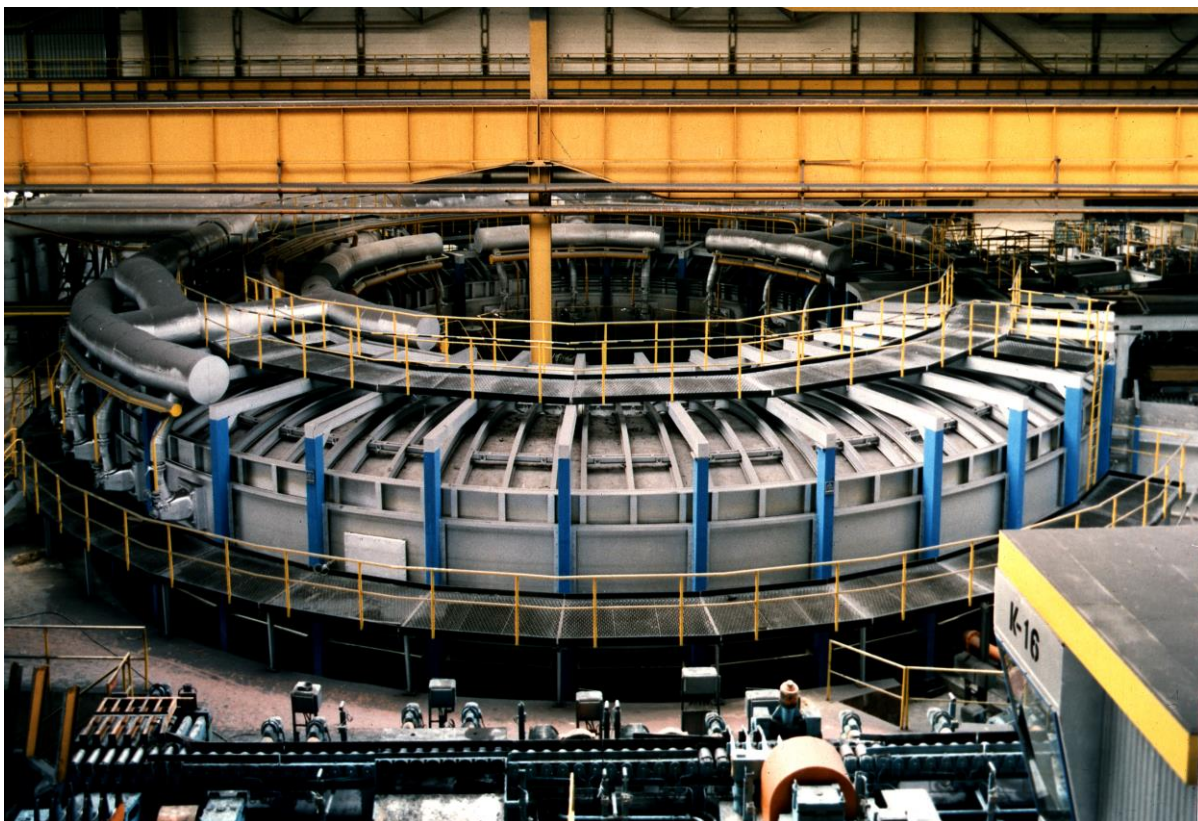
Nová karuselová ohrievacia pec v novej podbrezovskej valcovni vyhrievaná zemným plynom.
