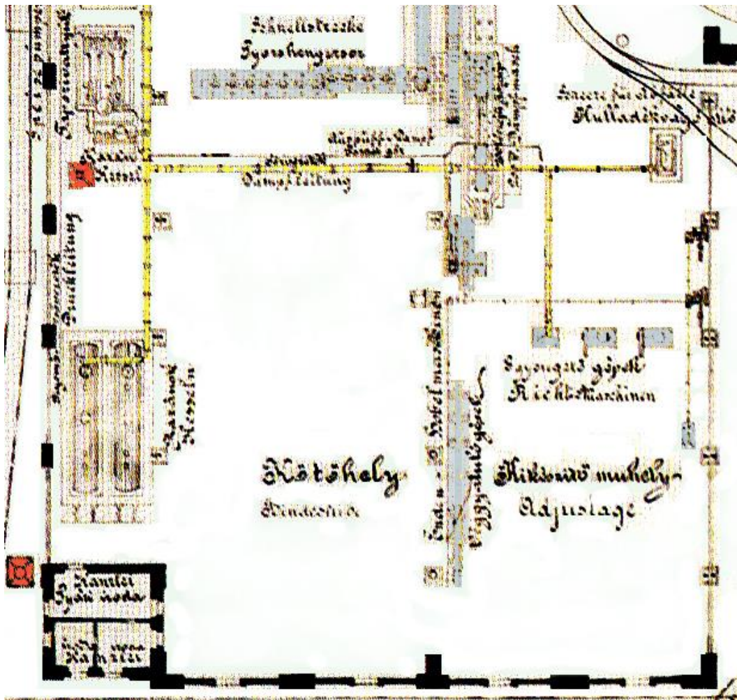
Výrez plánu podbrezovskej železiarne s dvojicou parných kotlov v spoločnej obmurovke ohrievacej uhoľnej pece na výrobu pary (celkom vľavo dole) aj s plechovým komínom (červená) s rozvodom pary (žltá) pre parný stroj valcovacieho poradia (modrá) vpravo hore a parných bucharov vpravo dole.
