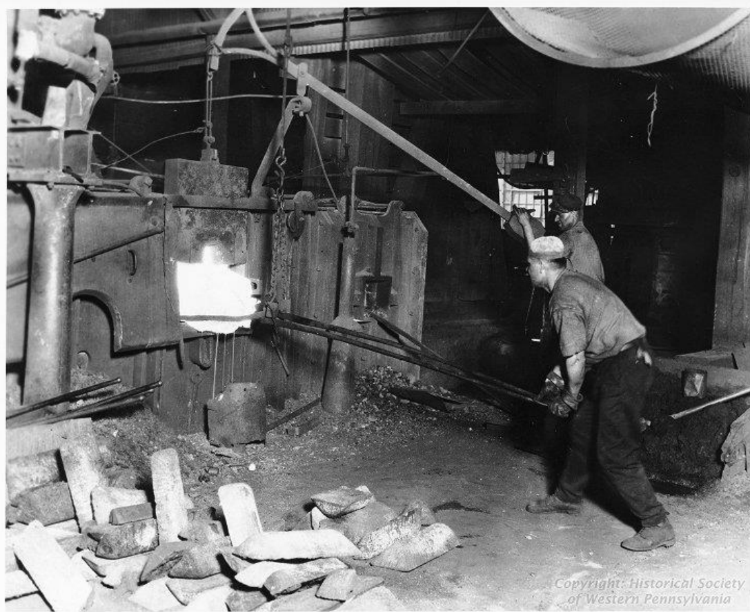
Vyberanie kujného železa z pudlovacej pece. Na zemi vľavo pripravená vsádzka húsok surového železa z vysokých pecí na niekoľko hodinové pudlovanie za účelom zníženia uhlíka.
