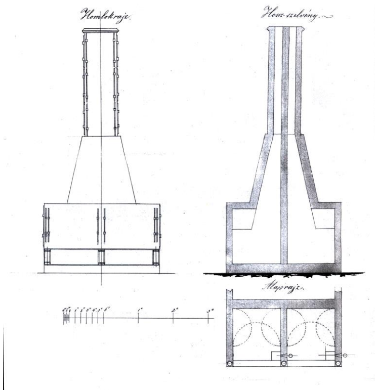
Dvojčitá vyhňa v spoločnej obmurovke z hámra v kostiviarskej.
