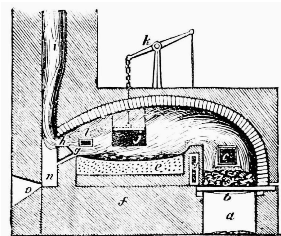
Princíp tavenia plameňom v pudlovacej peci: a. popolník a prívod vzduchu, b. liatinový rošt, c. otvor pre kľuftové drevo, e. nístej pece s okujami, f. murované telo pece, j. otvor pre vsádzku sur. Železa, pudlovanie a vyberanie kujného železa, i. odvod splodín, k. dvojramenná páka pre otváranie masívnych dvierok.
