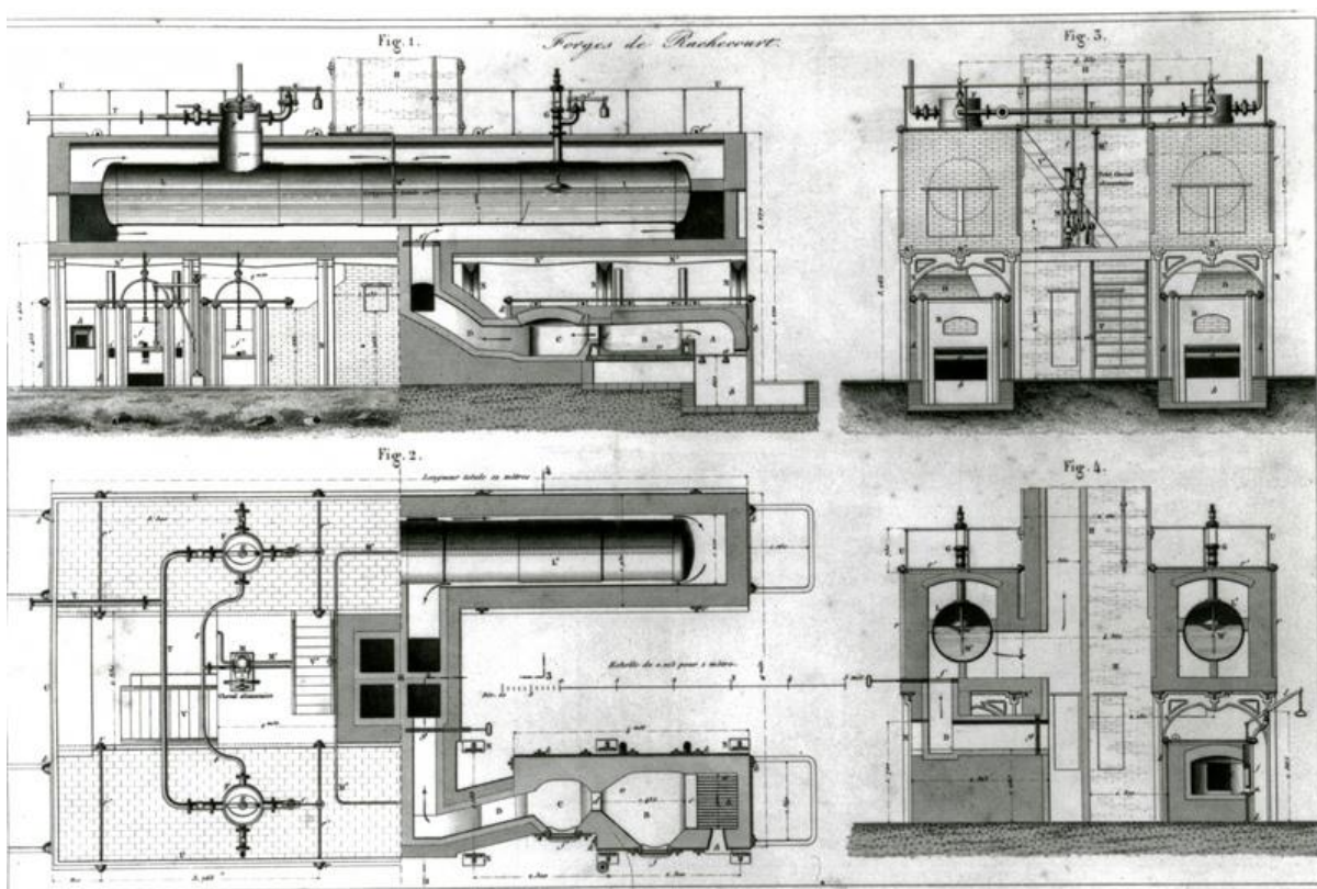
Príklad využitia odpadového tepla z batérie štyroch pudlovacích pecí na výrobu pary v kotloch umiestnených nad nimi.
