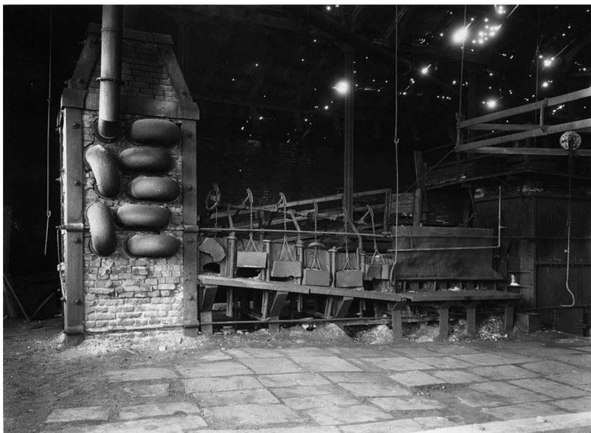
Ohrievacia pec s ohrievačom plynu v komínovej časti. Sklon pece umožňoval ľahší posun ohrievacích ingotov (deilov) pogaľovaním po naklonenej rovine smerom k výstupu z pece.
