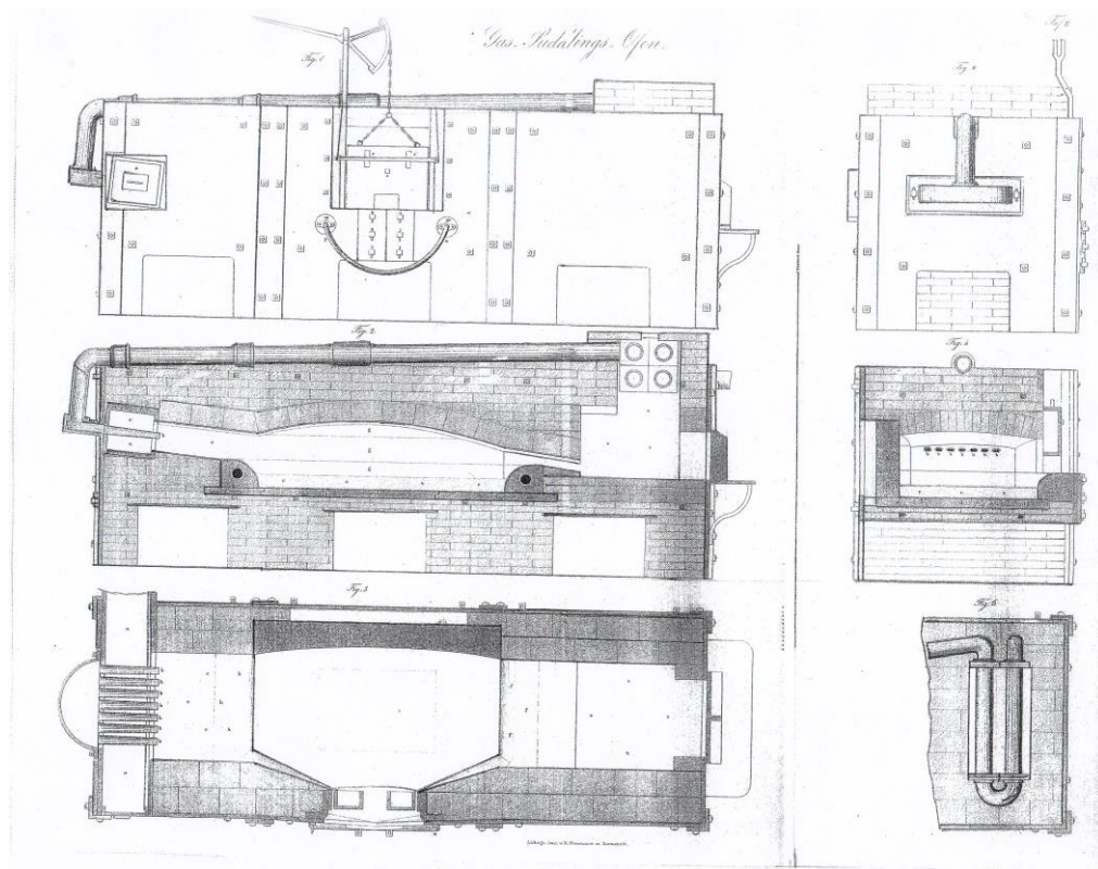
Zváracia pec na generátorový plyn s predhrevom.
