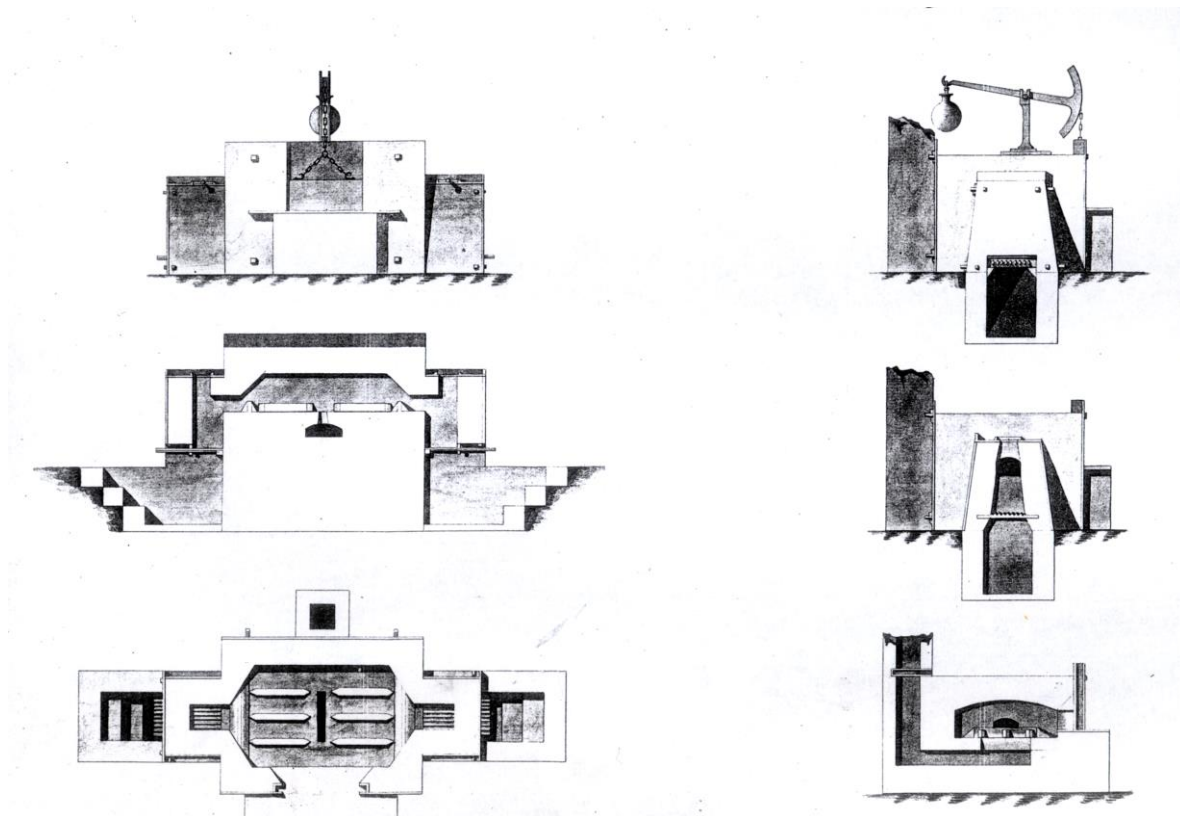
Plán ohrievacej pece vyhrievanej kluftovým drevom podobne ako v pudlovacích peciach.
