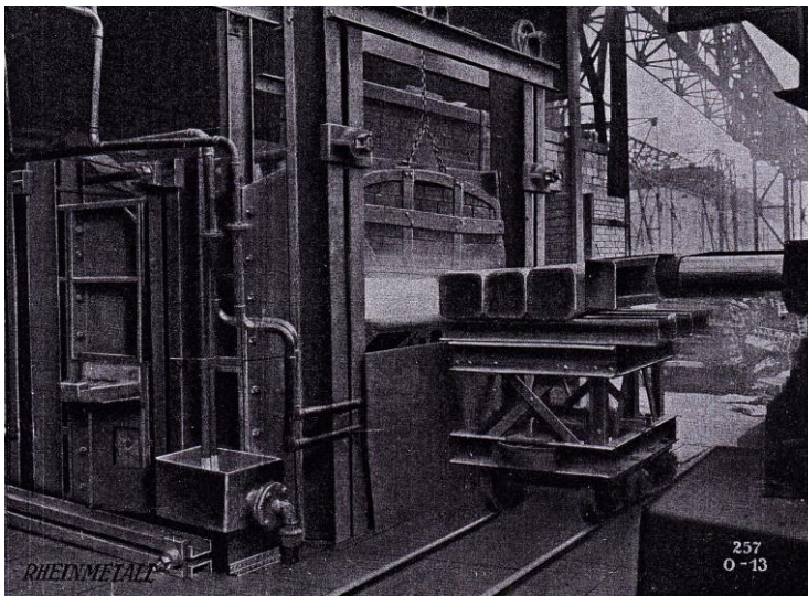
Narážacia pec na ohrev predvalkov so zasívacím zariadením v novej jemnej valcovni.
