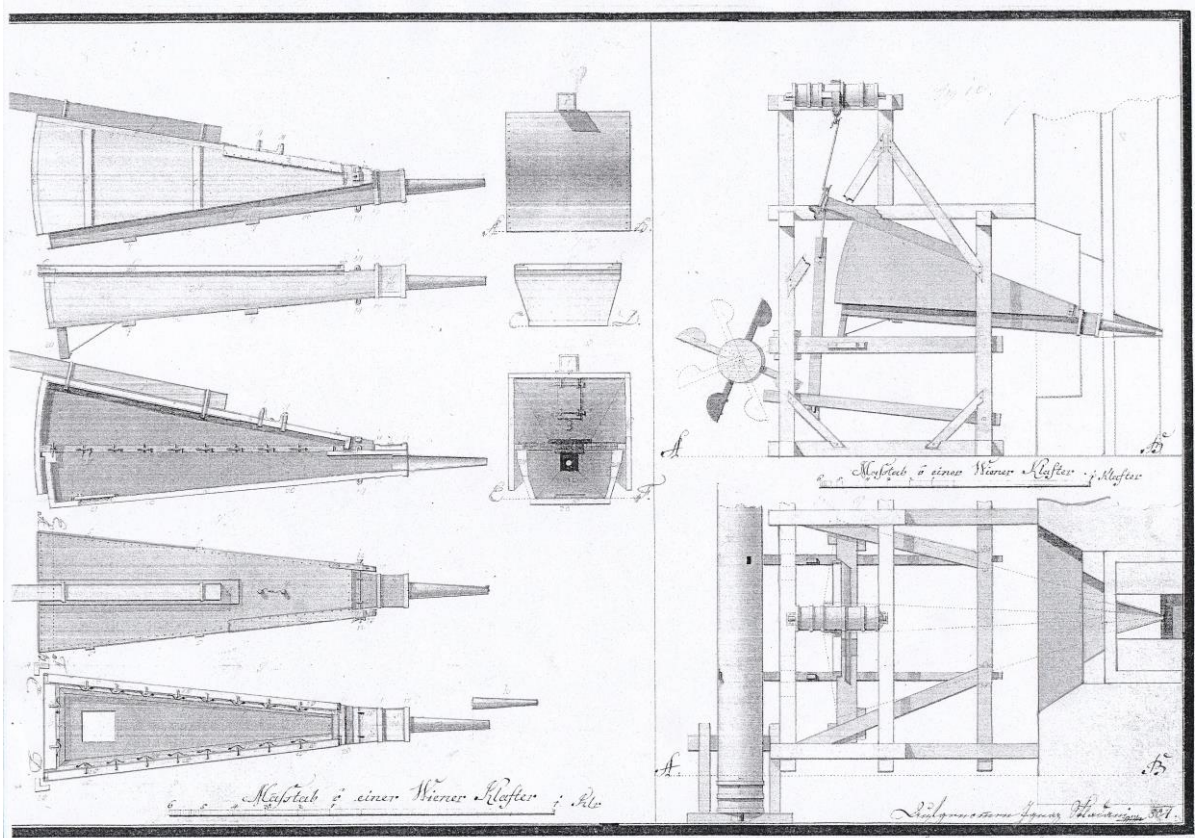
Plán truhlového dýchadla nahradzujúceho klasické kožené mechy..
