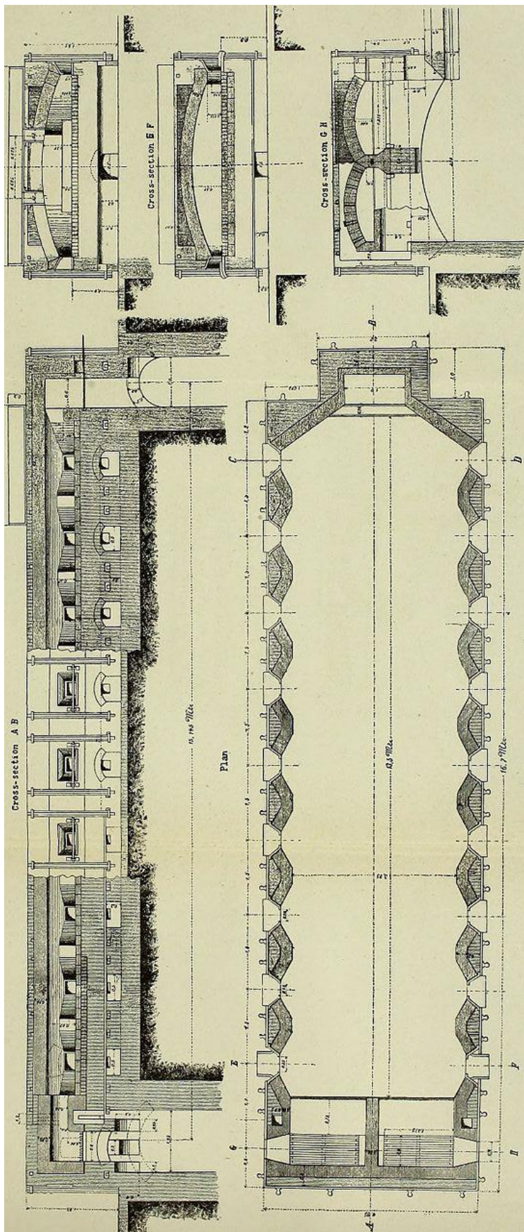
Plán ohrievacej pece ingotov na kamenné uhlie. Celkom dole dva roštové ohniská, hore komínová časť s usadzovačom popola a dechtu nazývaná kamra. Celkom hore rezy pece.
