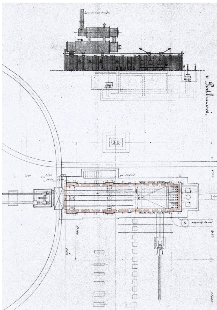
Narážacia pec v novej jemnej valcovni na generátorový plyn hore s kovovým rekuperátorom tepla na výrobu pary. Vľavo zariadenie na zasúvanie predvalkov zo železničného vozíka do pece so zásobovacou železničkou. Vpravo dole vyťahovací vrátok ohriatych predvalkov a valčekový dopravník k valcovaciemu poradiu.
