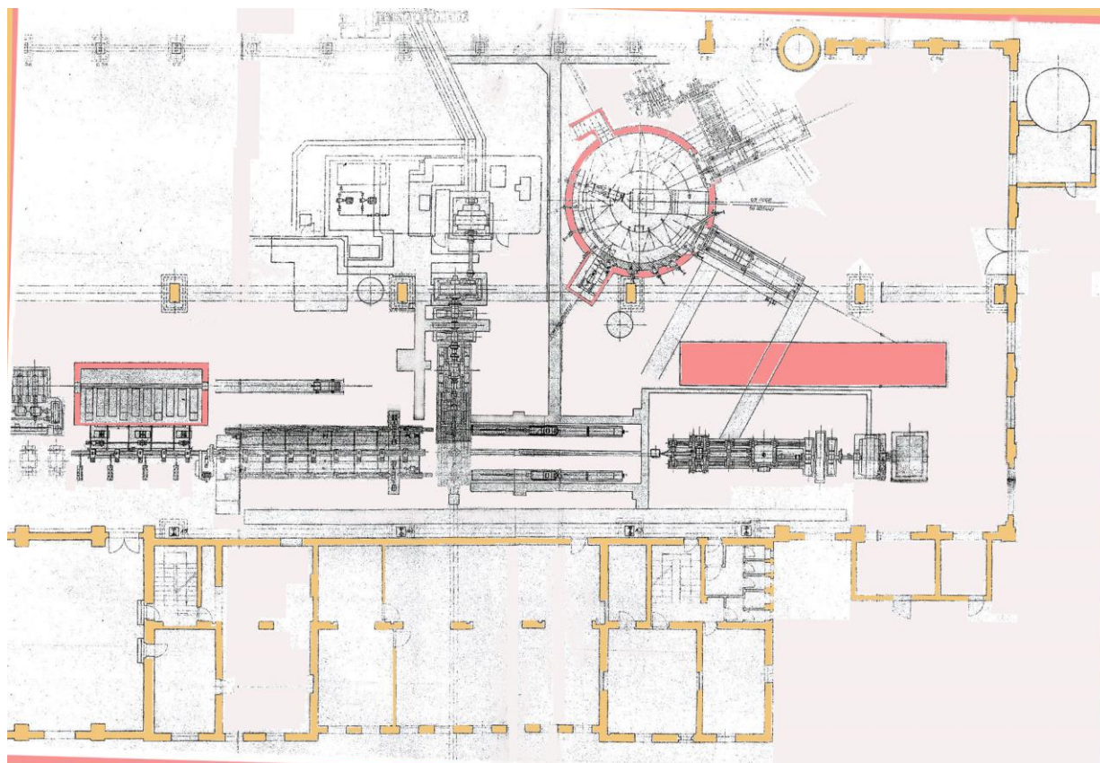
Prvá karuselová pec inštalovaná v 60. rokoch 20. storočia v starej rúrovni sa neosvedčila a robotníci až do jej zrušenia v 80. rokoch 20. storočia pracne posúvali valcové predvalky tyčami po smere ohrevu v starej pogaľovacej peci vyznačenej červene.
