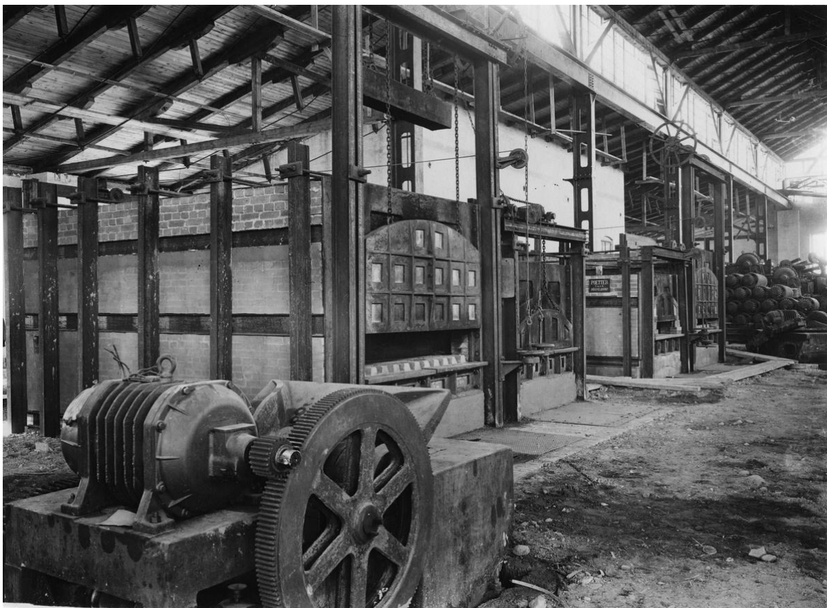
Žihacie a ohrievacie pece.
