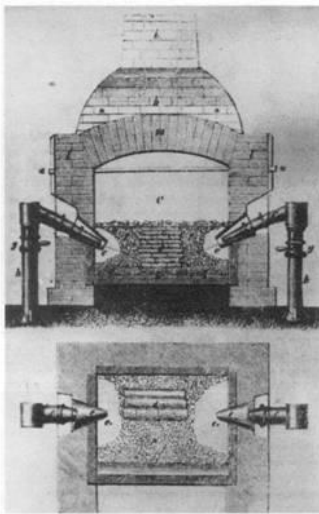
Hronecký typ vyhne s protíahými výfučňami
