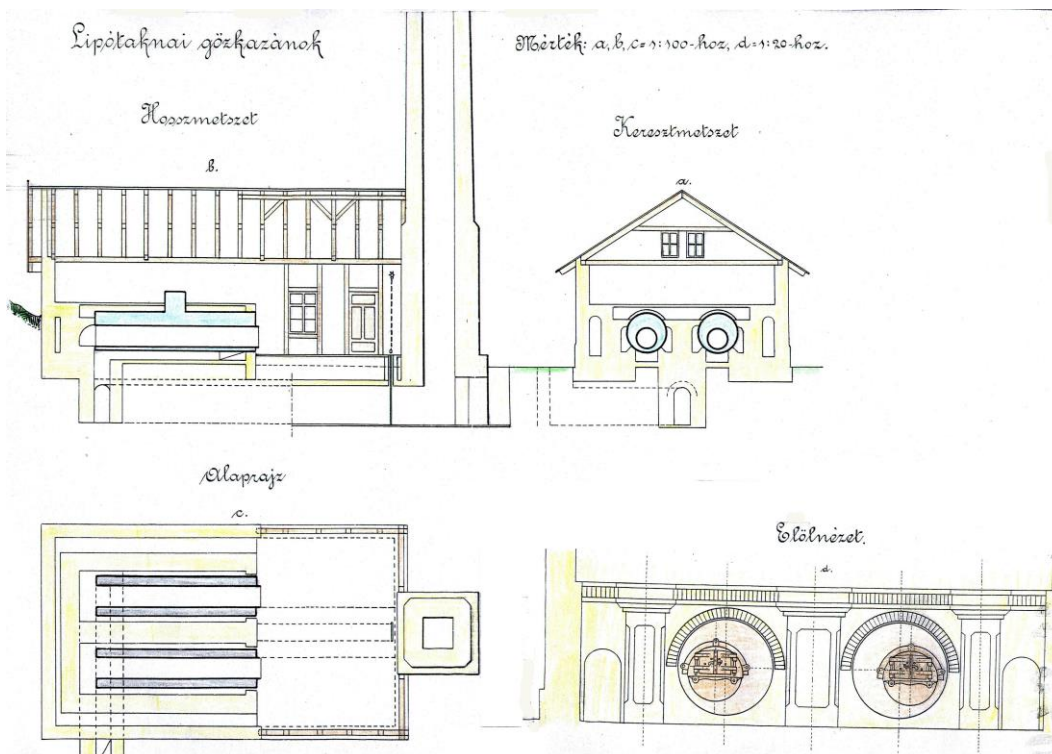
Konštrukcia kotla na preberacom protokole z r. 1914.
