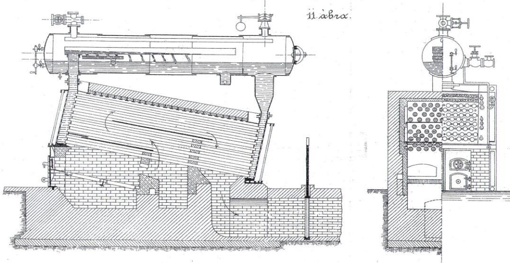
Kotel na výrobu pary značky Steinmüller.
