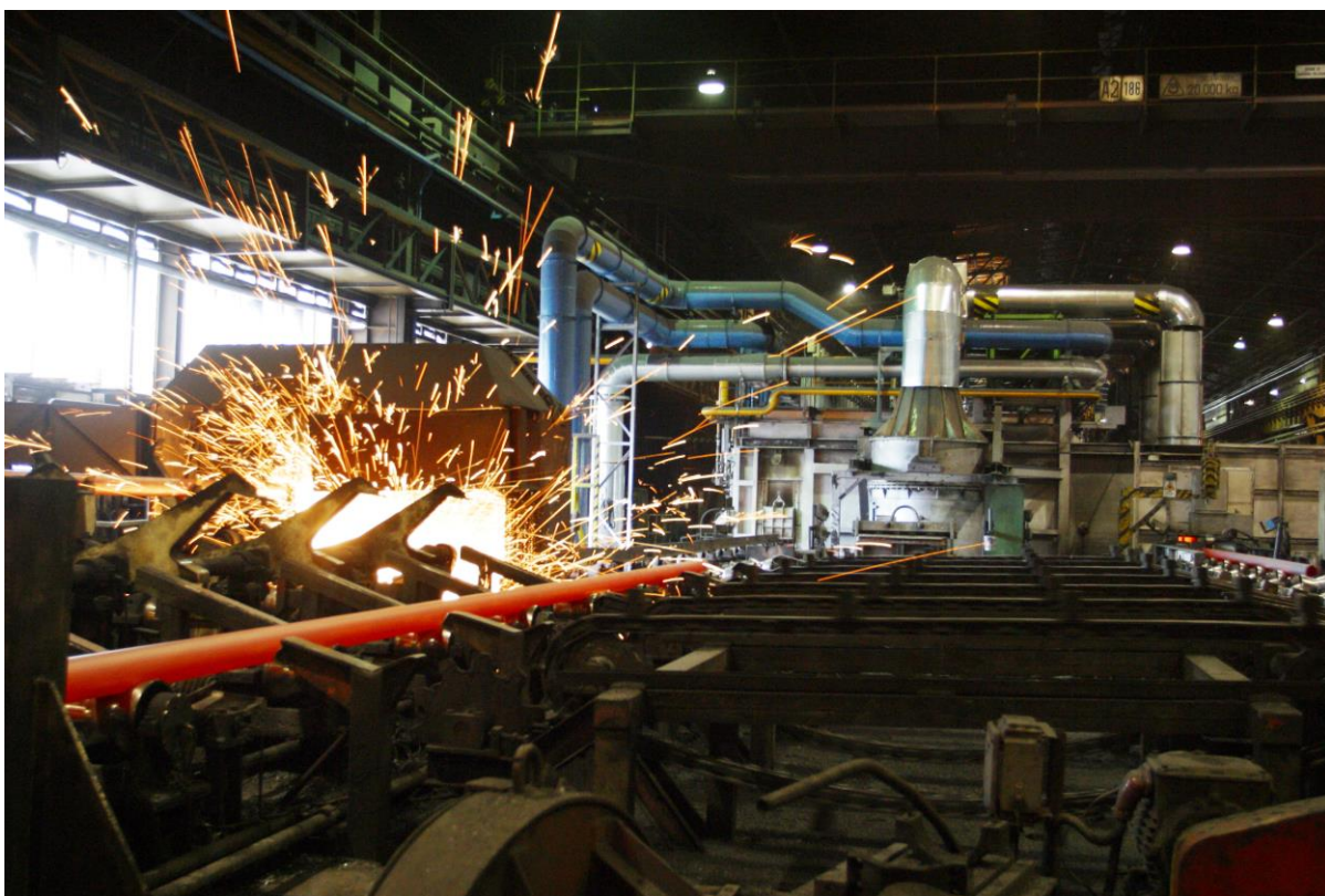
Ohrievacia kroková pec v novej rúrovni vyhrievaná zemným plynom.
