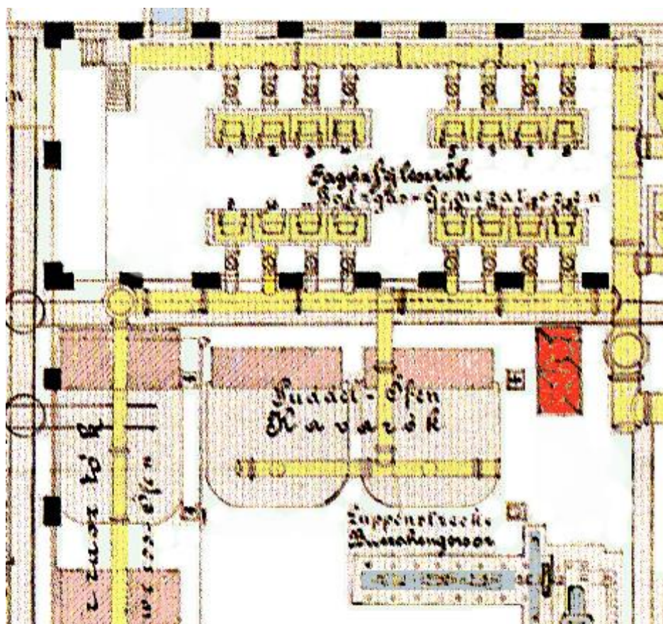
Výrez plánu podbrezovskej železiarne s dvojicou rekuperačných pudlovacích pecí (ružovo šrafované) uprostred s vyznačenou kamrou rekuperátorov základoch pecí (sivá) s vertikálnym prívodom generátorového plynu na ohrev a batériou uhoľných generátorov plynu celkom hore aj s plynovým potrubím (žltá). Vpravo dvojica plechových komínov (červená). Vľavo zväracie pece a celkom vpravo dole valcovacie poradie (modrá).
