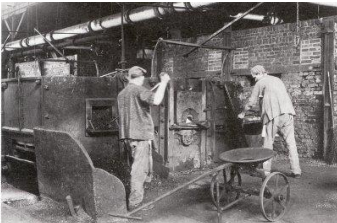
Prepravný vozík na presun žeravého kujného železa pod vykivacie kladivo (buchar).
