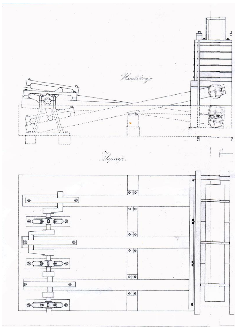
Batéria skriňových dúchadiel z hámra v Kostiviarskej neďaleko Baanskej Bystrici.
