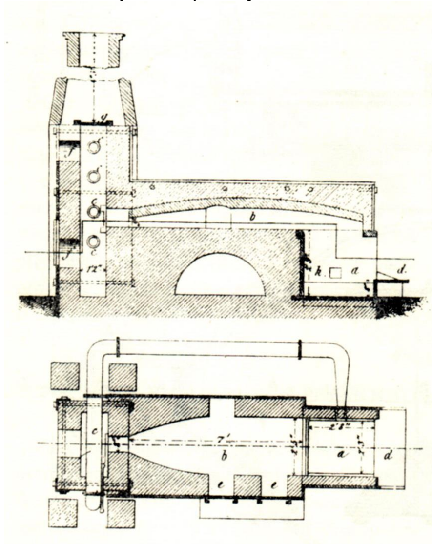
Comté vyhňa je priamym predchodcom pudlovacej pece. Na obrázku aj s ohrevom vzduchu.
