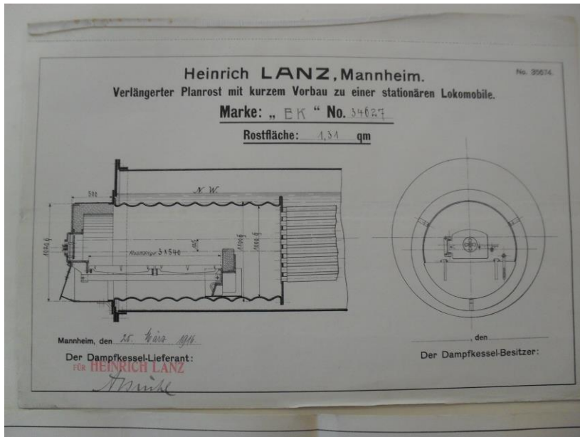
Konštrukcia kotla na preberacom protokole z r. 1914.
