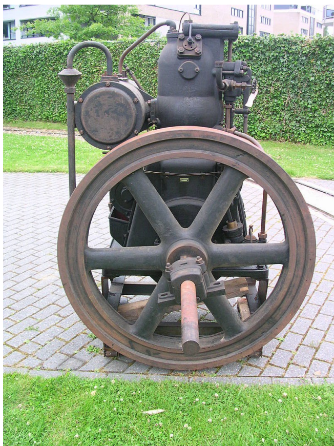
Motor na petrolejové výpary
