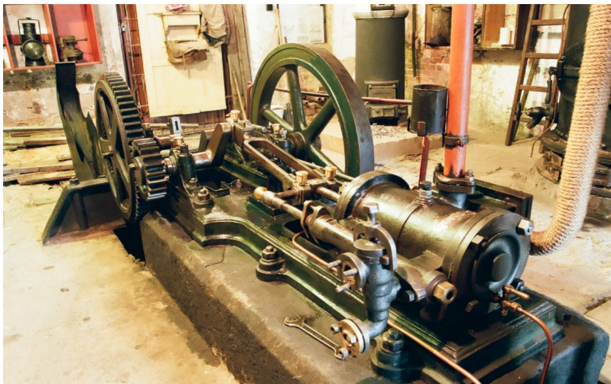
Pohľad na ležatý, jednovalcový, dvojčinný parný stroj.
