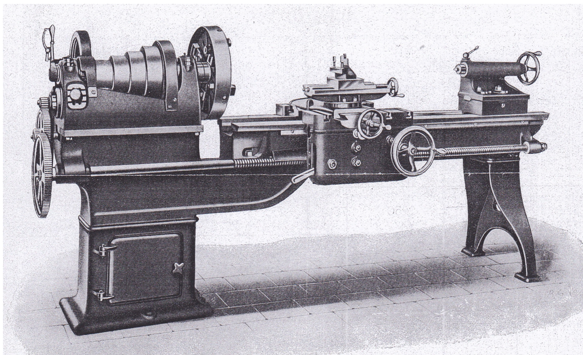
Sústruh s reguláciou otáčok zmenou priemeru remenice.
