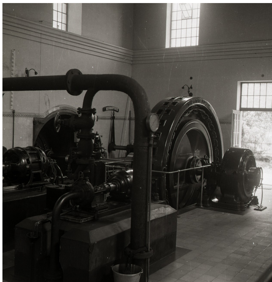
Interiér HC Lopej s generátorom a budičom.
