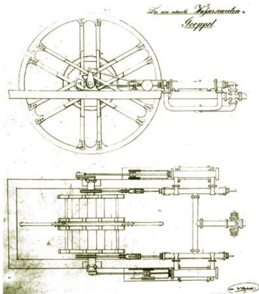
Plán vodnostlpcového ťažného stroja s navýjajím bubnom vľavo dvojicou ležatých valcov.
