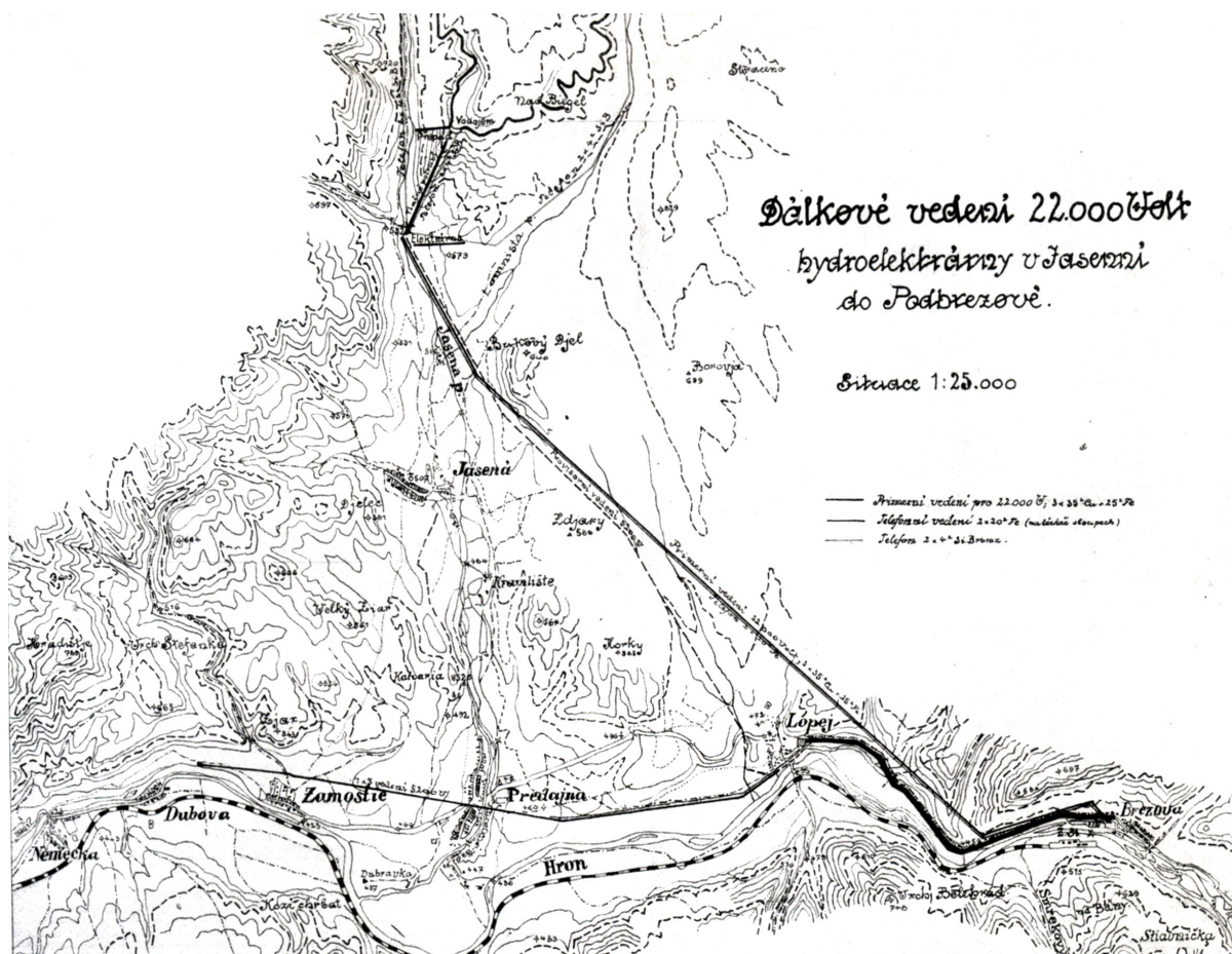
Plán diaľkového elektrického vedenia 22kV spájajúceho HC Jasenie (hore), s HC Dubová (vľavo) a HC Lopej s rozvodňou a transformovňou v Podbrezovej (celkom vpravo dole).
