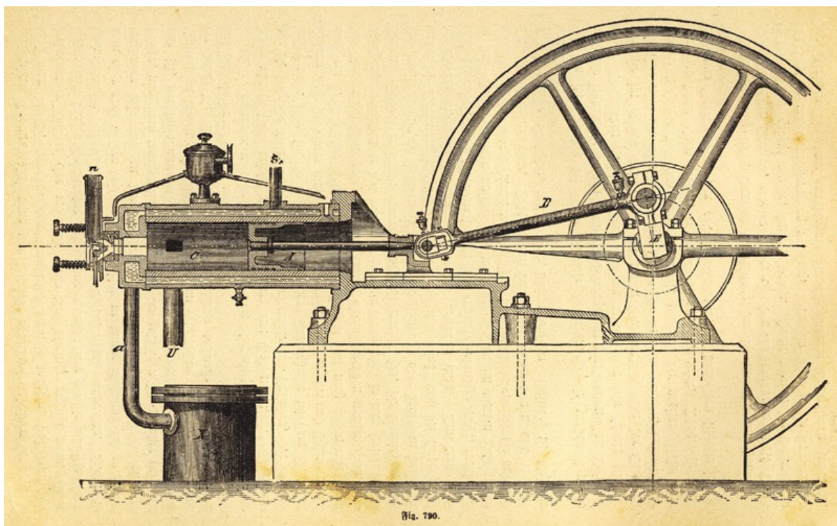
Tepelný motor s vnútorným spaľovaním petrolejových výparov
