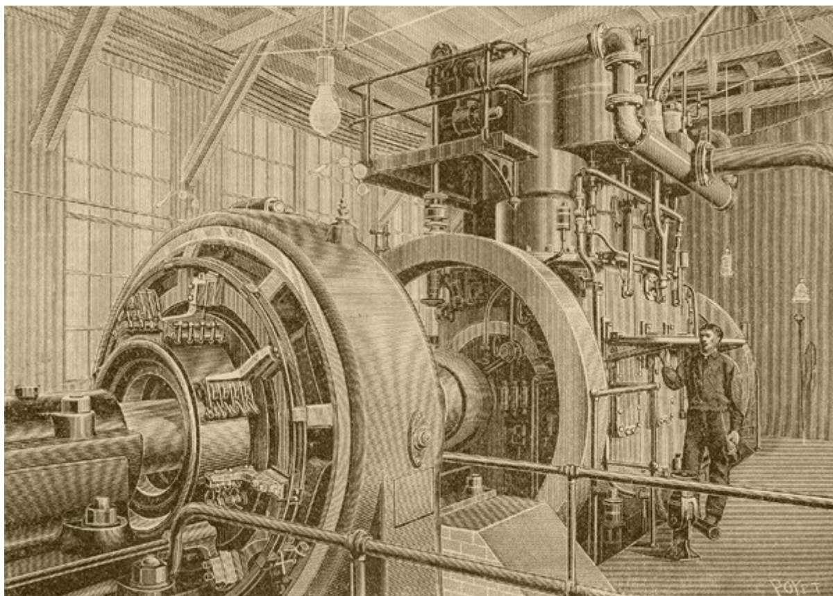
Plynový radový trojvalec na kychtový plyn pohánajúci generátor elektrickej energie.
