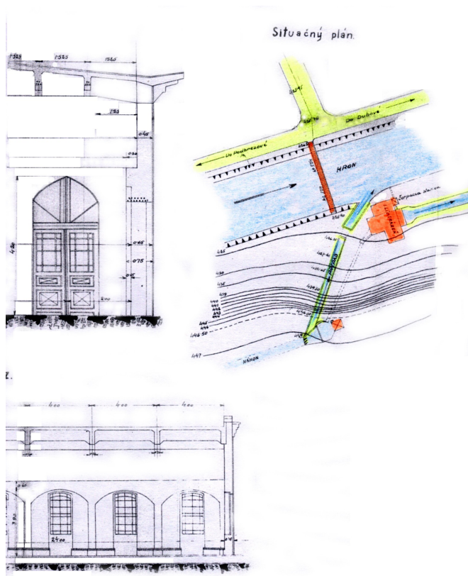
Situácia plan hydrocentrály v Dubovej s podzemným privádzačom o spáde 23m.
