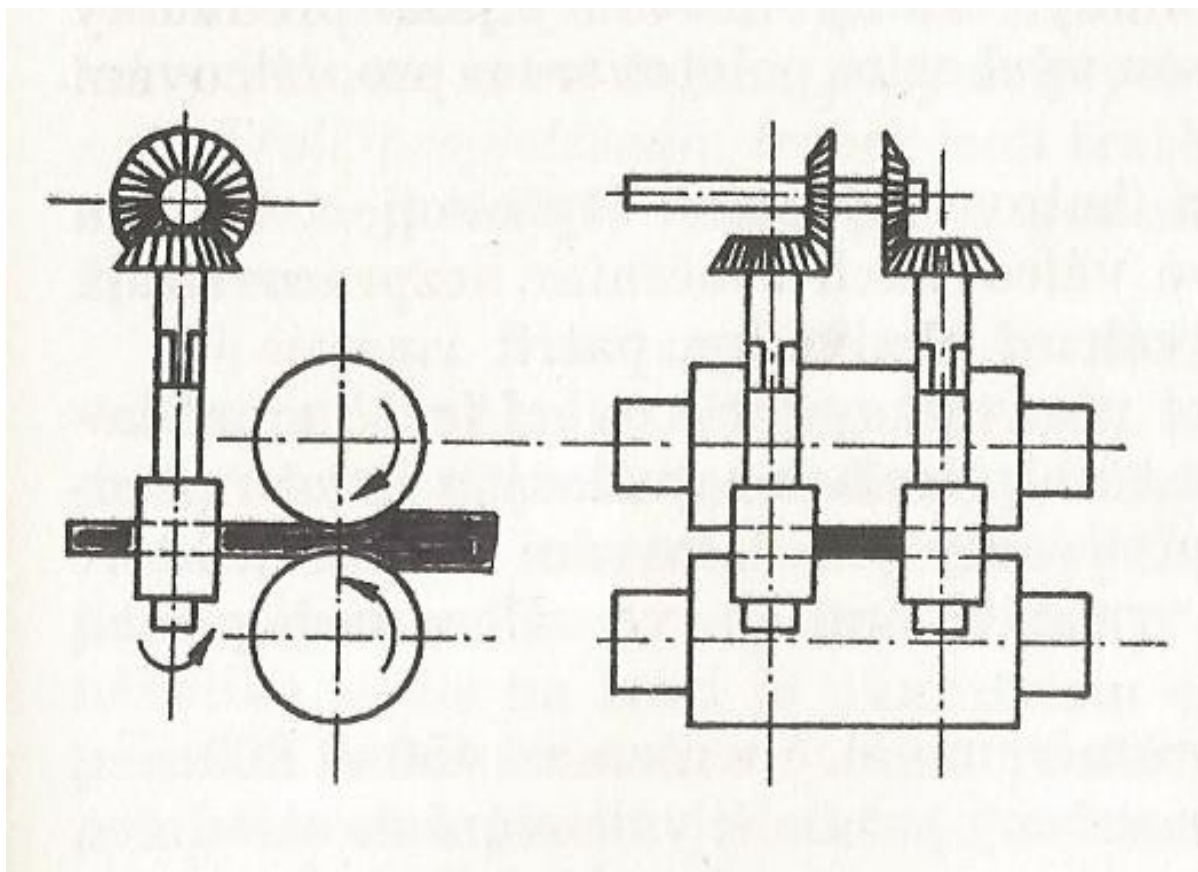
Princíp valcovania vo valcovacej stolici.
