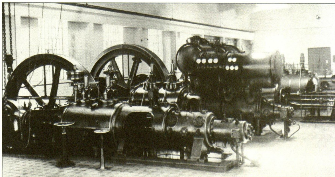
Strojovňa parnej elektrárne v Handlovej
