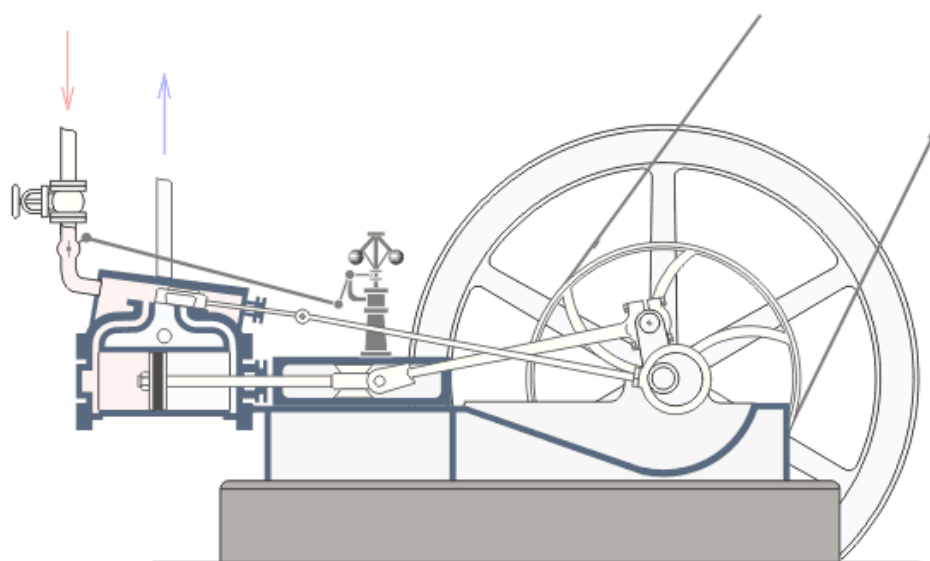
Rez najpoužívanějším ležatým parným strojem so zotrvačníkom.
