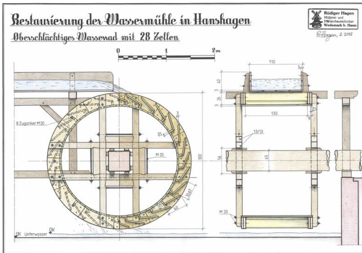
Drevená konštrukcia korčiekového vodného kolesa aj s vodným žľabom pre vodný mlyn.
