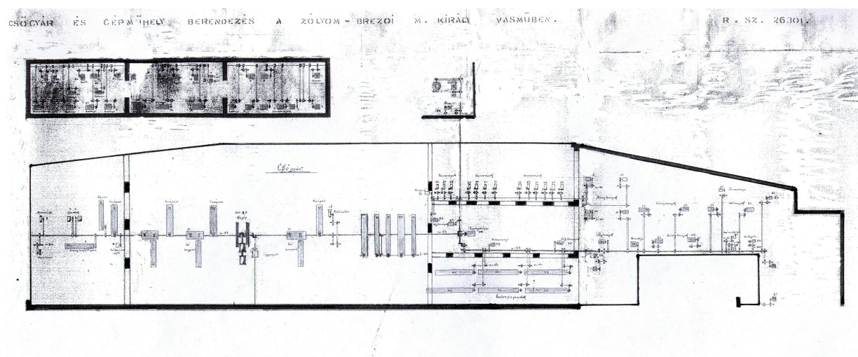
Schématický plán starej rúrovne s vyznačeným tandemovým parným strojom (vľavo).
