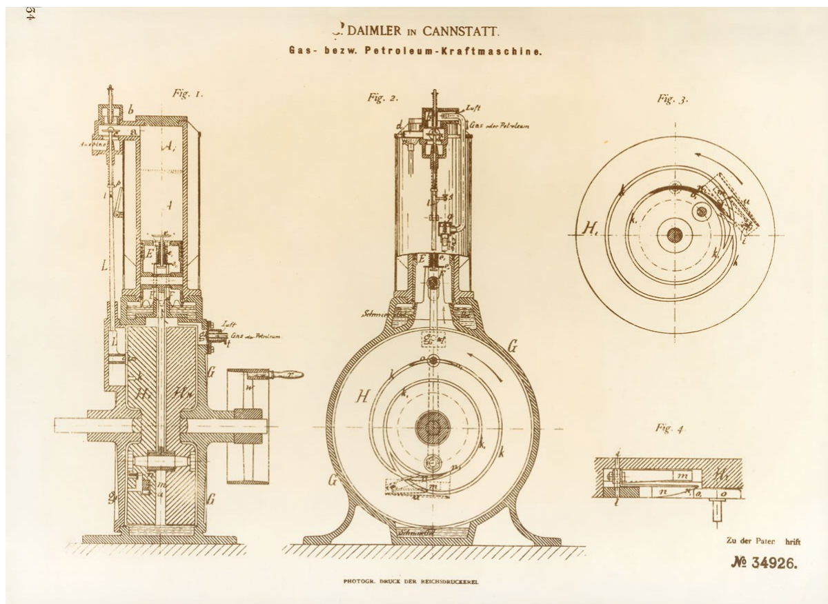
Jednovalcový spaľovací motor Daimler a Cannstatt.
