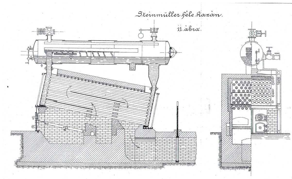
Kotol na pevné palivo na výrobu pary pre pohon parných strojov. Vďaka prúdeniu (cirkulácii) ohrievanej vody v rúrkach sa jej ohrev zintenzívnil a zvýšila účinnosť kotla.
