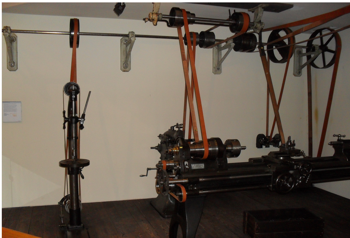
Sústruh poháňaný centrálnym motorom transmiou ktorý nahradil vodné koleso a neskôr aj parný stroj.
