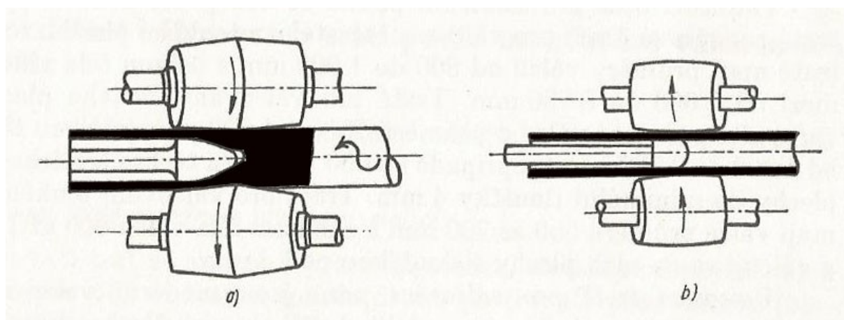
Princíp dierovacej stolice a) hladiacej stolice b) pri valcovaní rúr.
