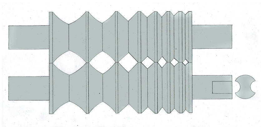
Typy valcov na valcovanie tyčovej ocele.
