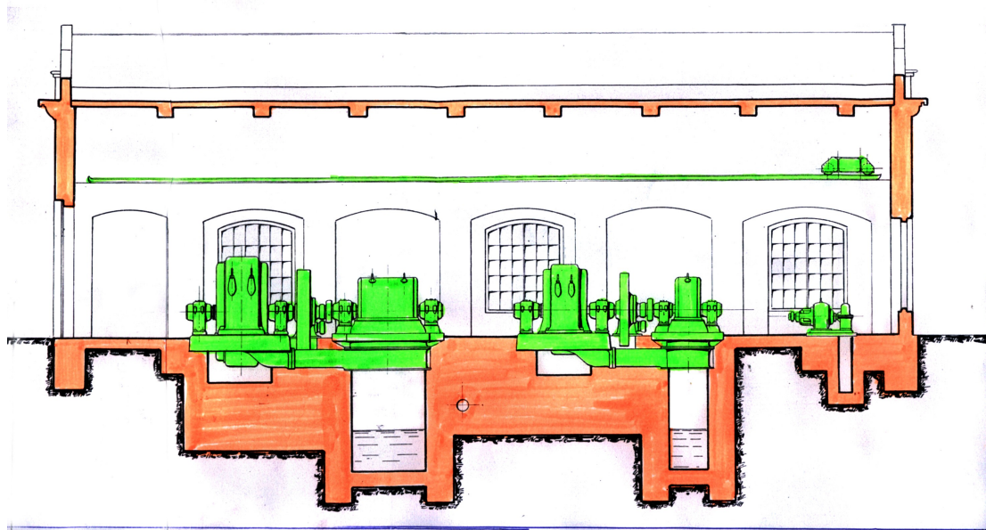
Rez objektom elektrárne v Jasení s dvojicou hlavných Peltonových turbín (vľavo dvojčíta) a jednej pomocnej (vpravo). Pod turbínami sa nachádza odpadový vodný kanál.
