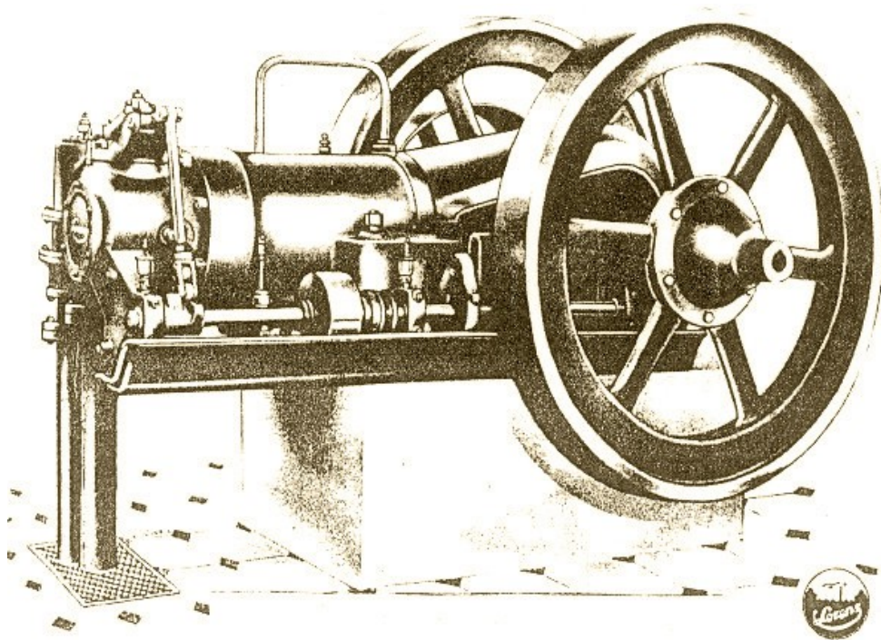
Stabilný jednovalcový, dvojčinný parný stroj s ležatým valcom s ventilmi a vačkovým hriadeľom na betónovom základe sa už začína podobat' prvým spaľovacím motorom.
