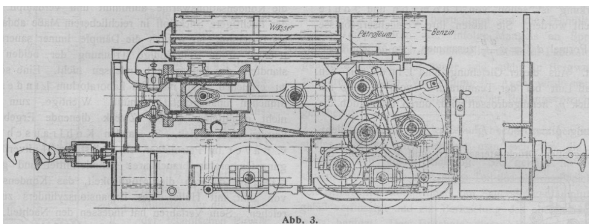
Spaľovací motor na výpary petroleja v banskej lokomotive
