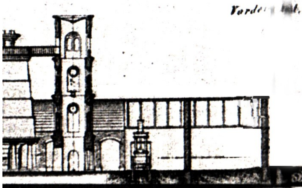
Valcove dýchadlo spojené netradične zvisle s parným piestom ako tandem (hore parný valec dole objemnejší valec dýchadla). V hroneckej hute boli tri takéto samostatné dýchadlá.
