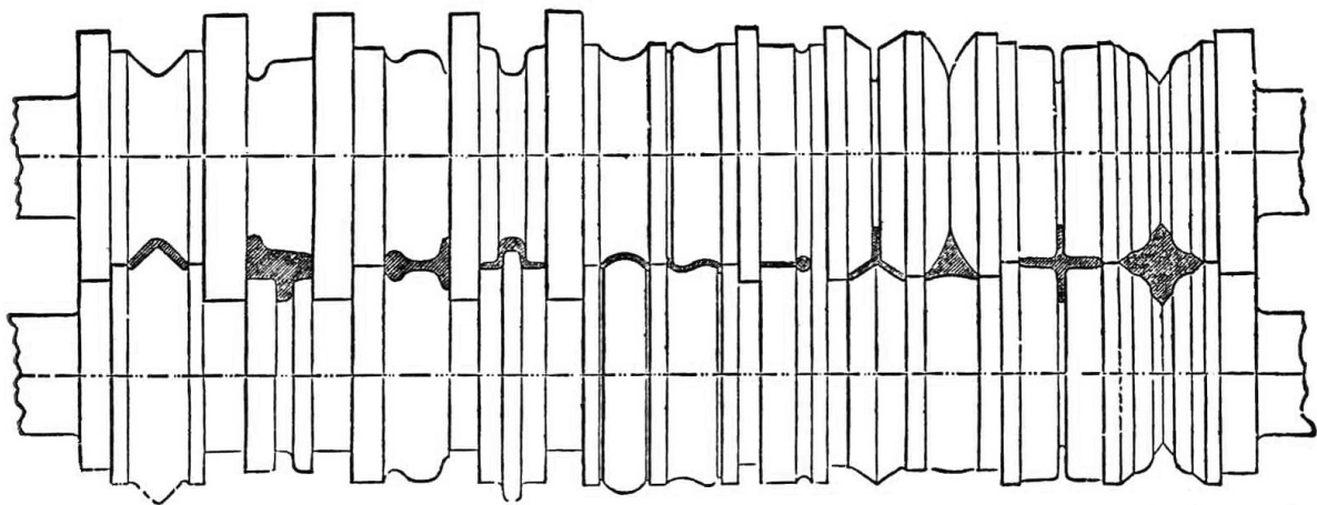
Ukážka páru valcov univerzálnej stolice pre valcovanie profilov vyznačených čierne.
