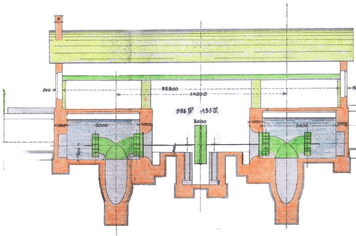
Priečný rez hydrocentrálou v Podbrezovej na pôvodnom vodnom náhone a odpadovom kanále s dvomi dvojčíťmi Francisciho turbínami na spoločnom hriadelí s generátorom uprostred.
