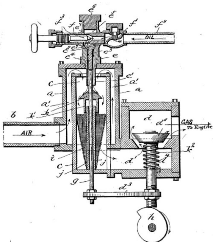
Prvý karburátor na miešanie zápalnej (výbušnej) zmesi vzduchu a výpary petroleja.
