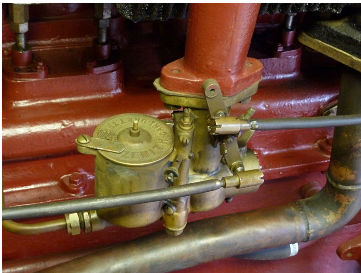
Pohľad na benzínový karburátor
