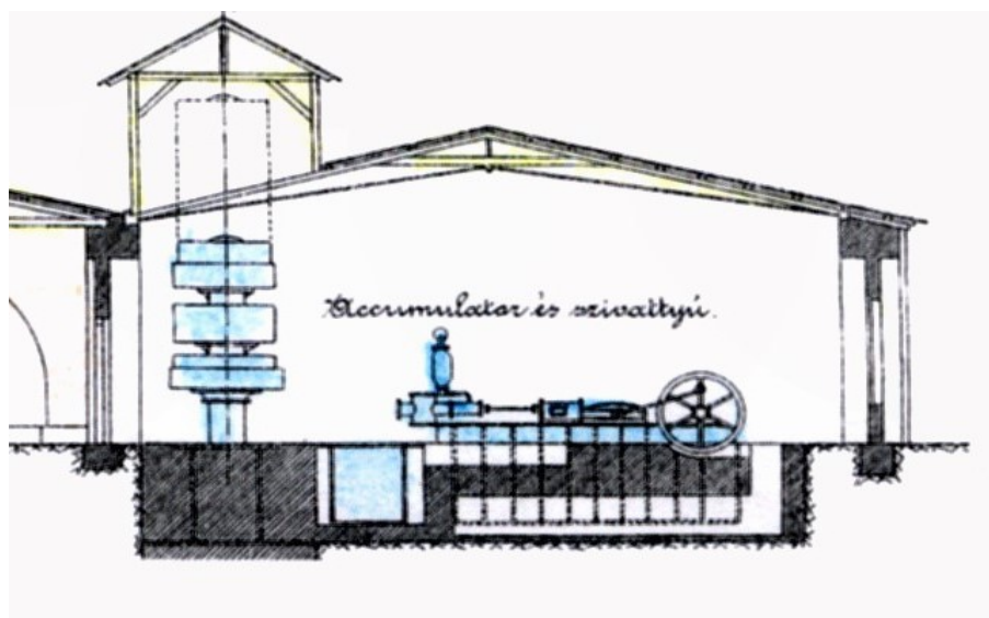
Detail plánu SM oceliarne s parným strojom v tandeme s čerpadlom.
