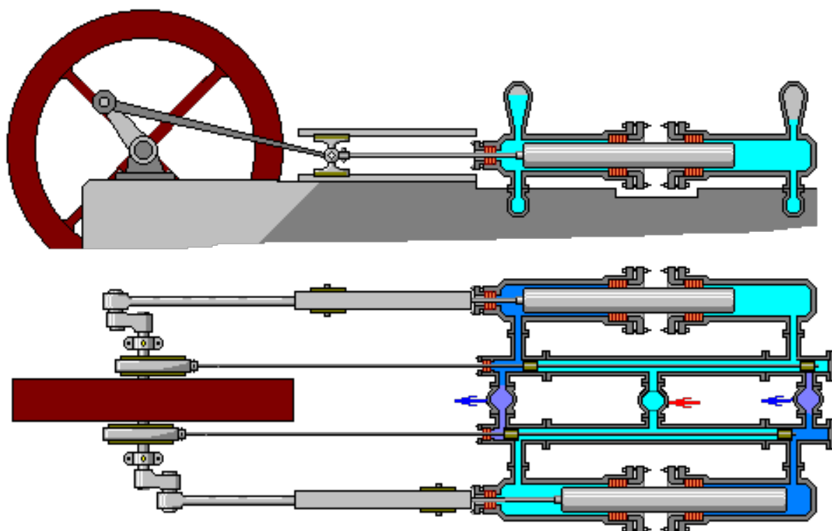
Princíp vodnostlpcového stroja kde tlaková voda(zelená, červený vstup) tlačí cez valcové šupátko (ako v parnom stroji) na piesty. Odpadová voda odteká voľne (modrá, modrý výstup).
