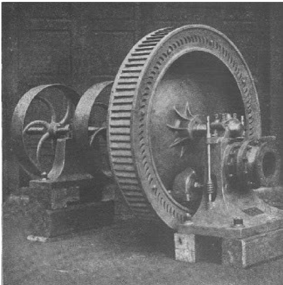
Giraldotova vodná turbína patrí medzi najstaršie vodné motory nahradzujúce vodné koleso s už vyššou účinnosťou. Podbrezová mala päť takých turbín.
