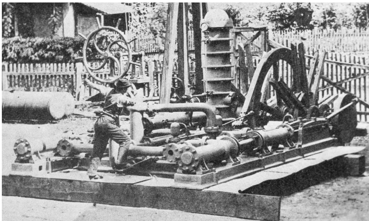
Vodnostlpcový ťažný stroj postavený v Hodruši v šachte Hill v roku 1800
