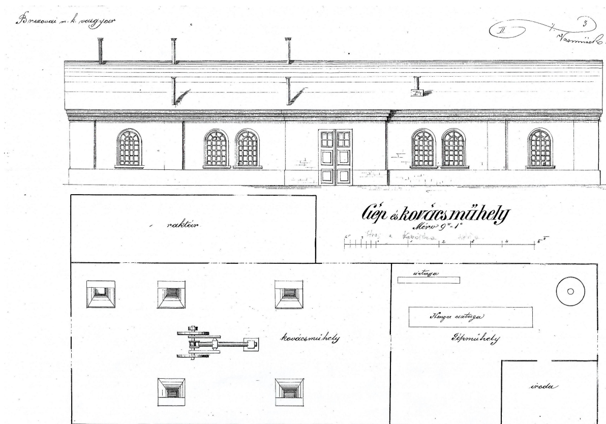
Plán kováčskej dielne s vykúvacím kladivom poháňaný parným strojom transmissiou z rúrovni
