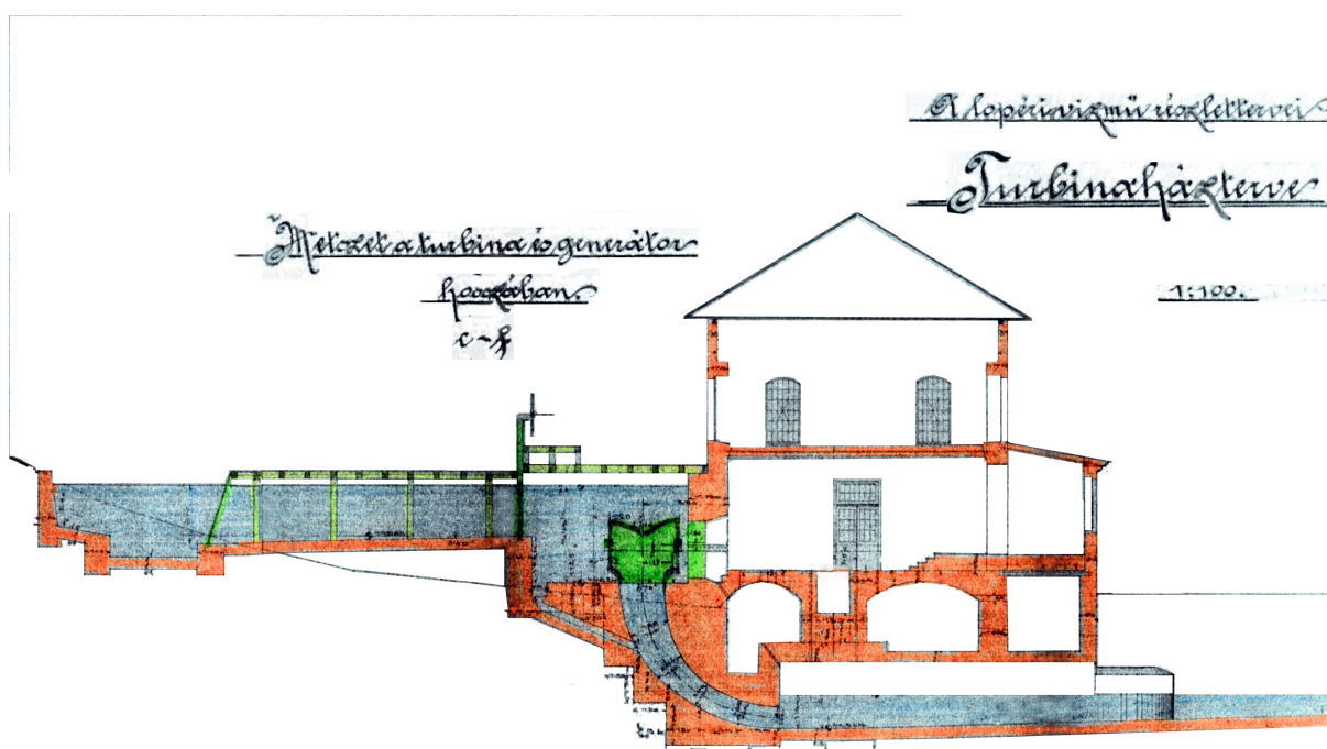
Pozdĺžny rez hydrocentrálou Lopej.
