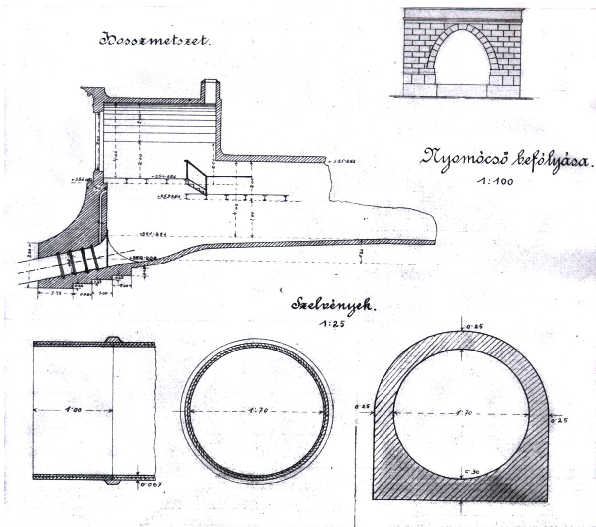
Vtokový objekt privádzača s tlakovým potrubím pre HC Piesok.
