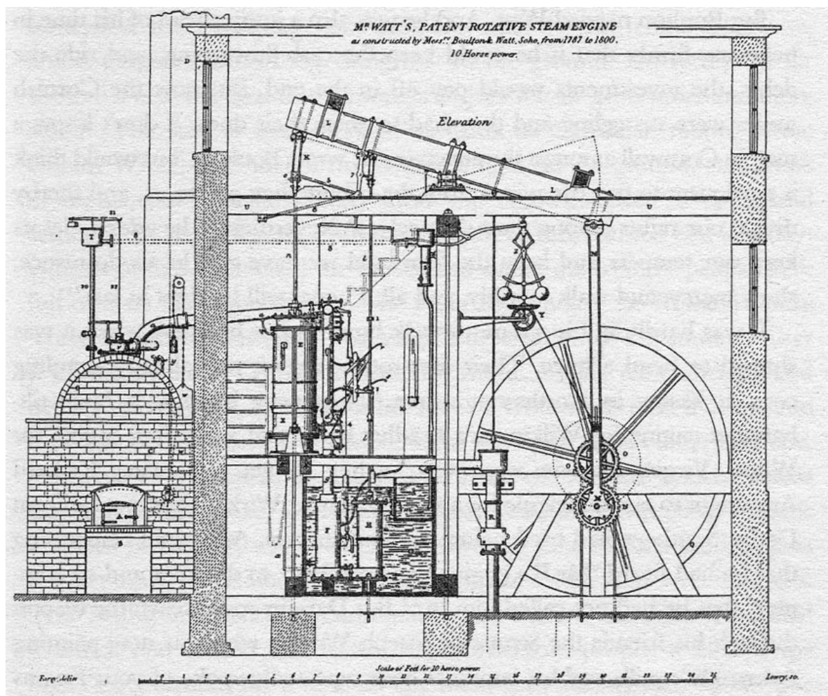
Plán Wattovho transmisného parného stroja už s Wattovým odstredivým regulátorom otáčok
