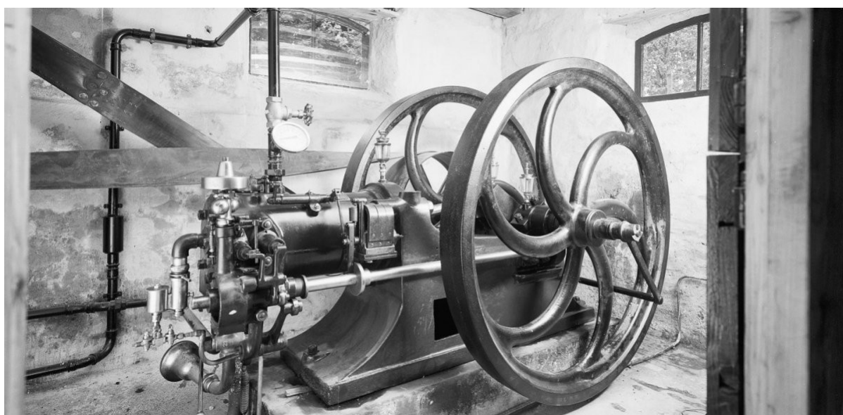
Spaľovací motor s elektrickým zapáľovaním na benzín alebo petrolej.
