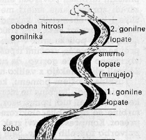
Sl. 4 Shema dvovenčne Curtisove turbine (postopno izkoriščanje hitrosti)
