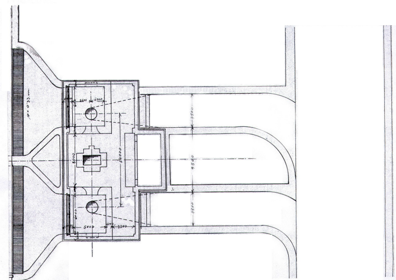
Vodná elektráreň v Podbrezovej pozdĺžny rez a pôdorys.
