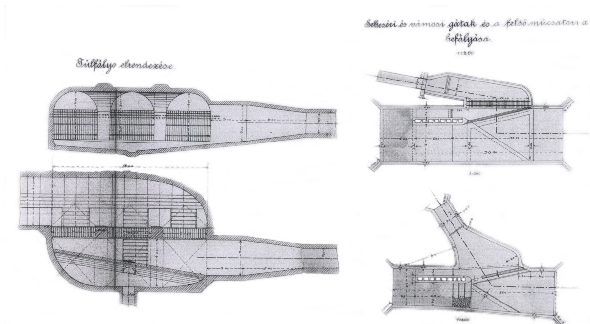
Podzemná komora s česlicami na sedimentáciu piesku s prepadom a haťové telesá.
