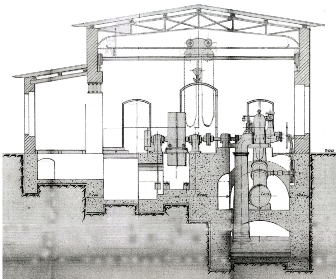
Priečny rez HC Piesok s generátorom a turbínou, pod ňou s tlakovým privádzačom a odpadovým kanálom.
