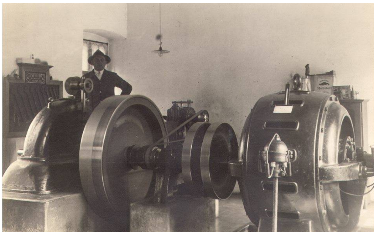
Peltonova vodná turbína so zotrvačníkom, regulátorom otáčok a generátorom elektrického prúdu určená pre veľké vodné spády a malé prietochné množstva.
