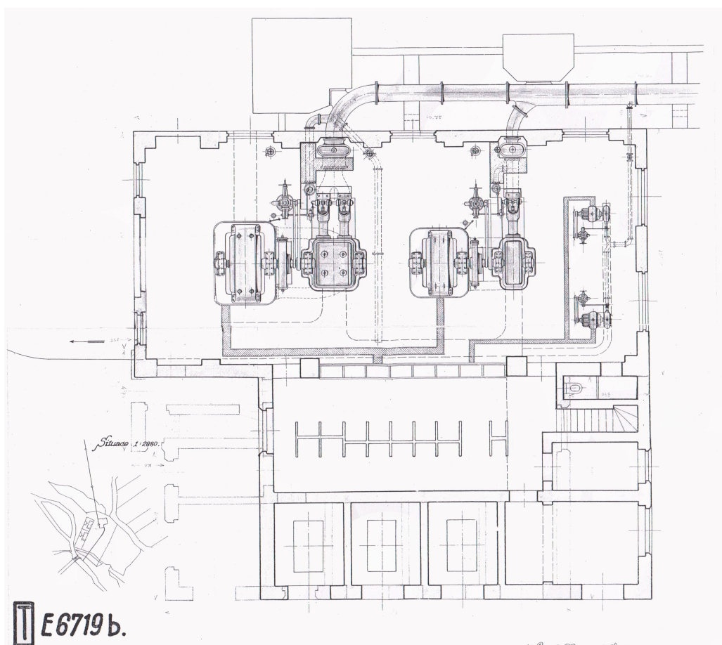
Plán elektrárne s dvojicou hlavných peltonových turbín a dvojicou malých turbín vpravo.
