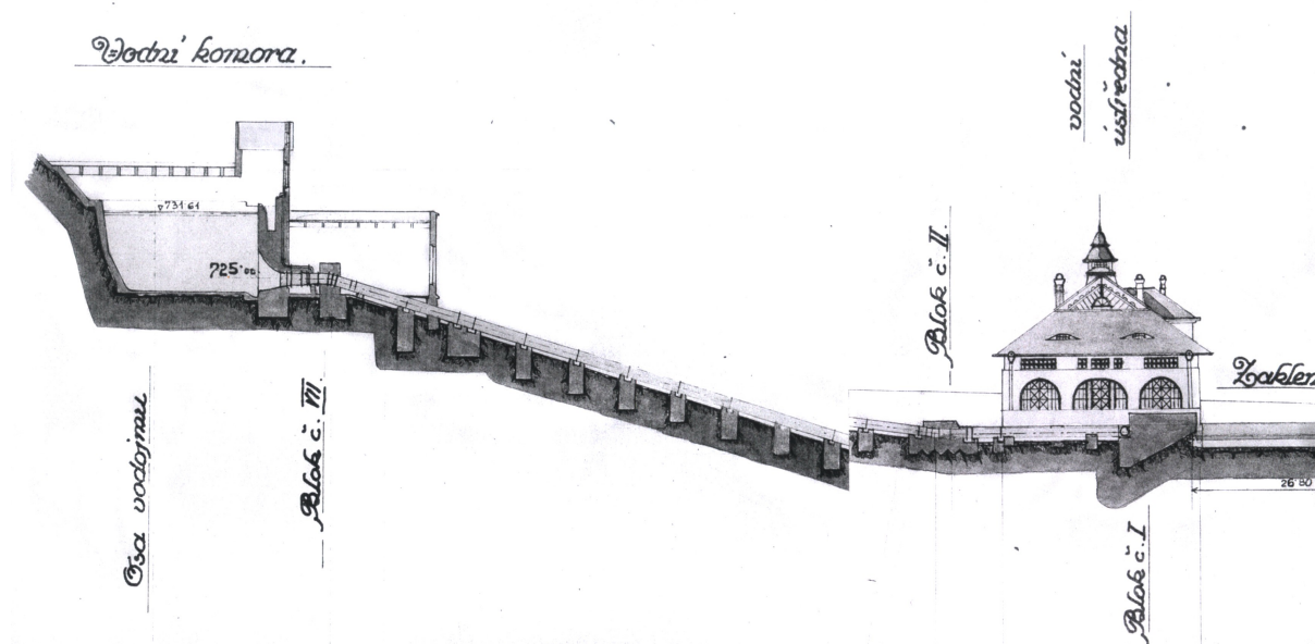
Rez vtokovým objektom (vľavo) a privádzačom do elektrárne (vpravo).
