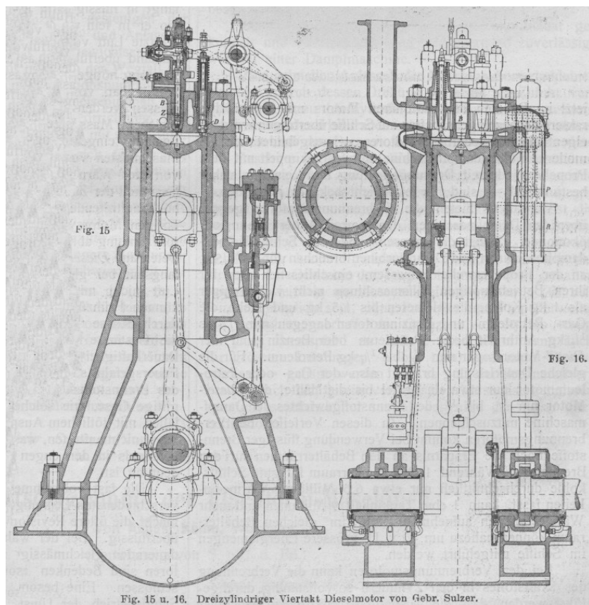
Spaľovací motor s priamym vstrekom paliva do valca.
