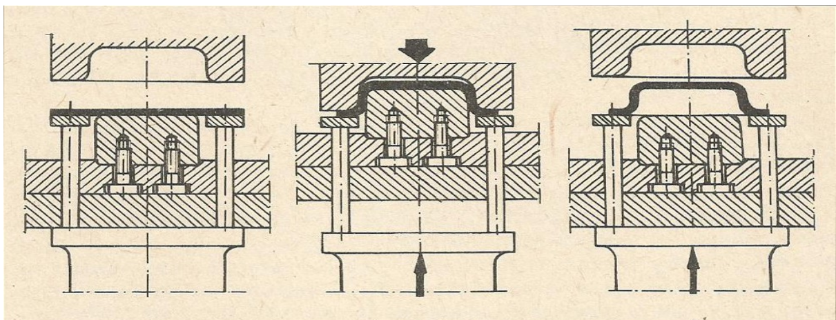
Princíp tvárnenia plechu lisovaním: vľavo plech položený na ťažníku a pridržiavačoch, v strede ťahanie plechu šmykadlom zhora s jeho brzdením pridržiavačmi, vpravo pridržiavače zodvihnú výlisok z ťažníka.
