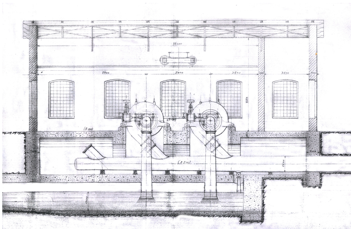
Pozdĺžny rez HC Piesok s dvojicou špirálových Francisciho turbínami.
