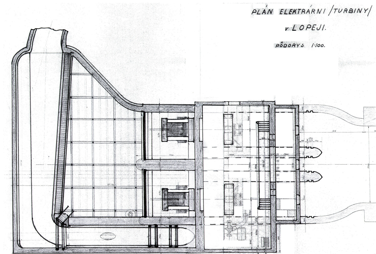
Plán HC Lopej s privodným kanálom vľavo hore s česlicami a odpadovým kanálom vpravo.
