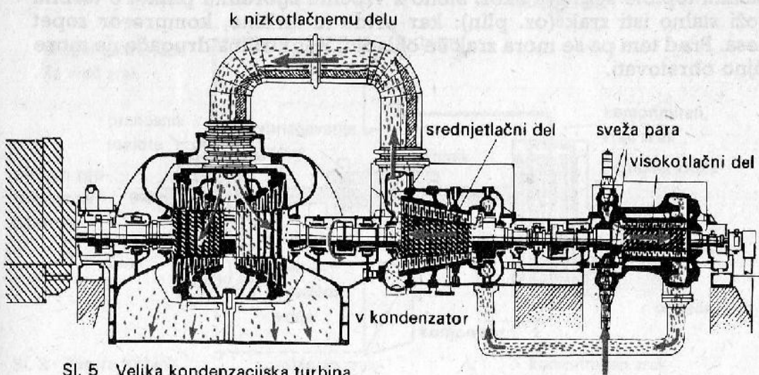
Sl. 5 Velika kondenzacijska turbina
