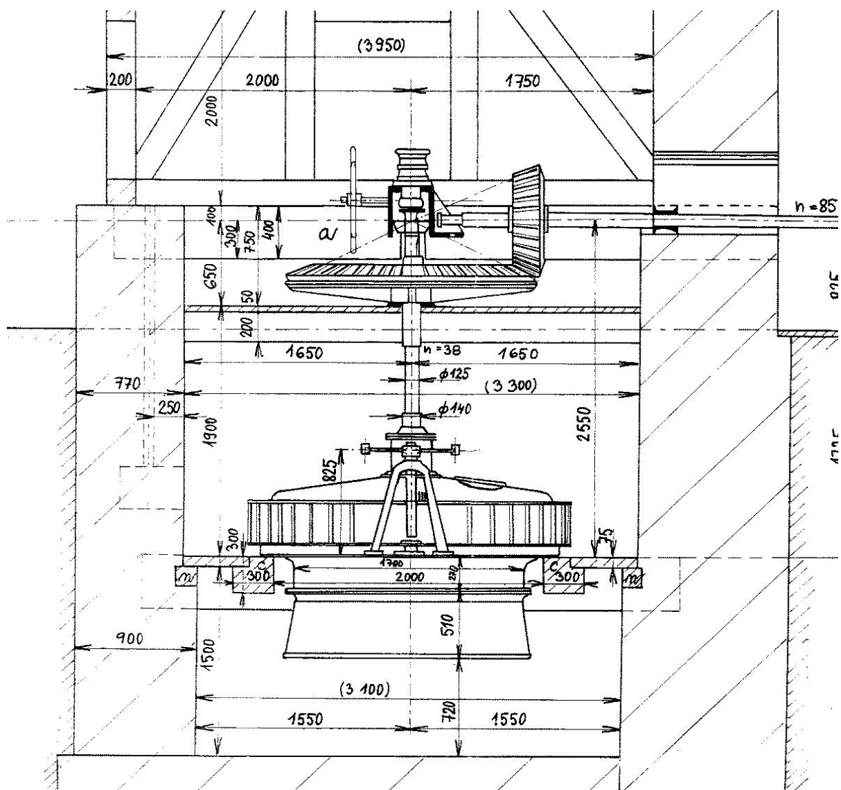
Girardotova turbína uložená vertikálne v šachte s uhlovým ozubeným prevodom hriadele.
