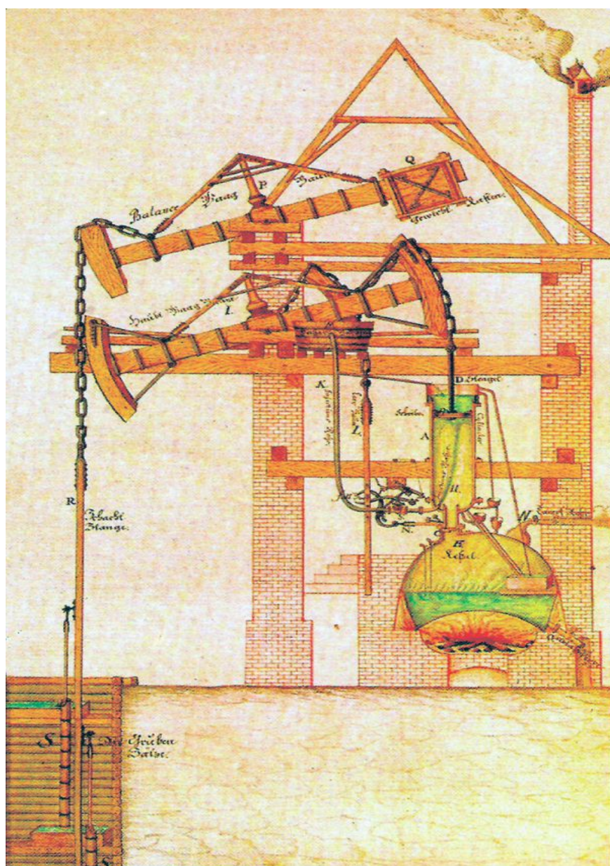
Ohňový atmosférický stroj na čerpanie banských vôd postavený v Novej Bani v roku 1722 ako prvý na Európskom kontinente. O desať rokov neskôr postavili ďalšie dva v Štiavnických Baniach.
