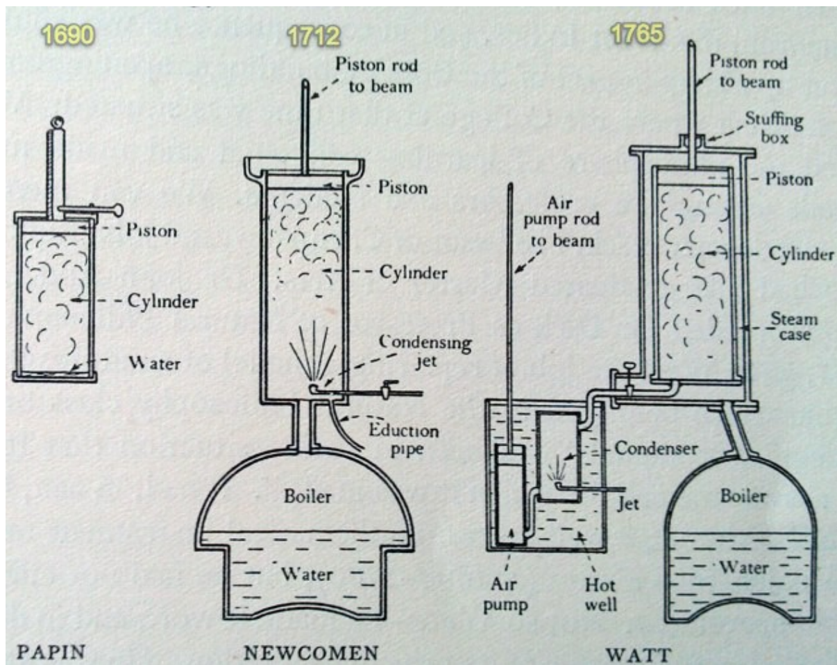
Princíp atmosferického a Wattovho stacionárneho parného stroja
