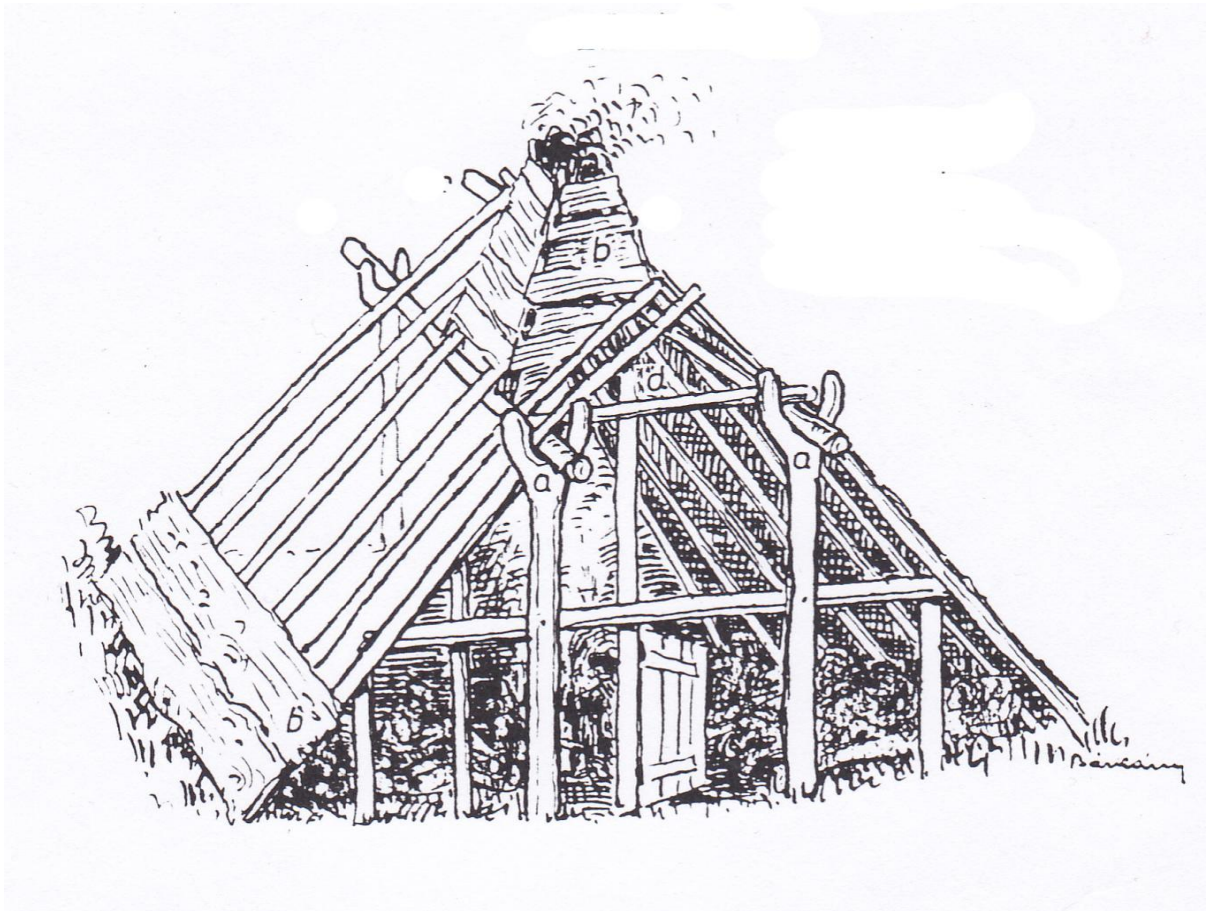
Obr. 6. Konštrukcia uhliarskej koliby s použitím krytiny z čerstvej kôry smreka alebo jedle.
