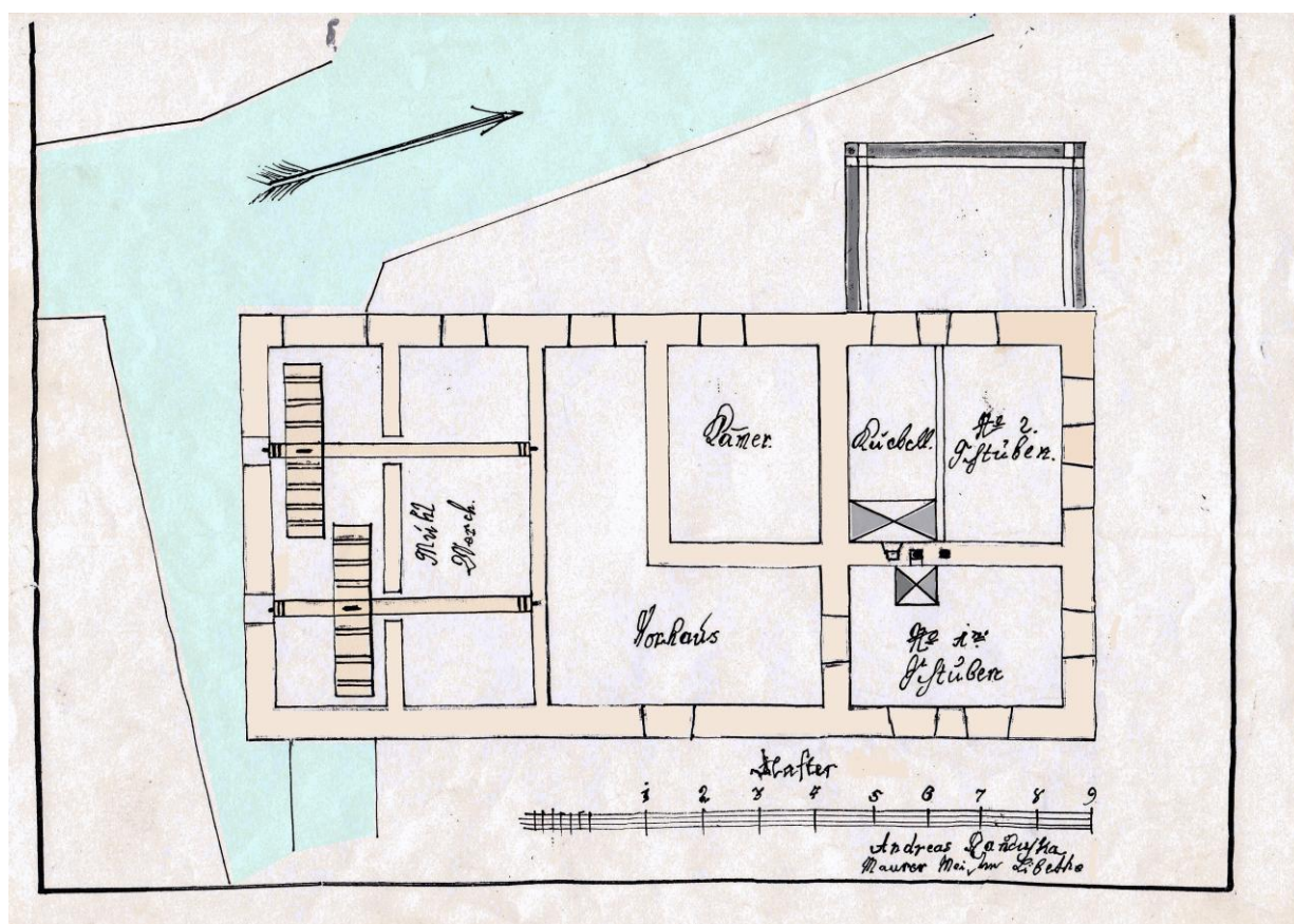
Obr. 21. Plán komorského dvojkamenného mlyna so skladovou sýpkou v Hronci.
