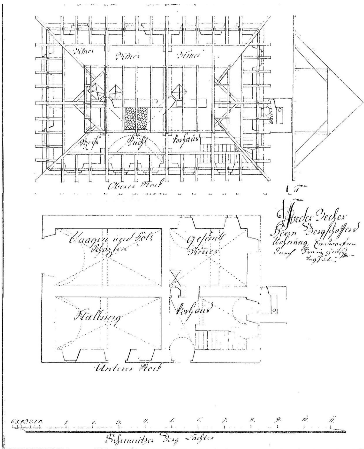
Obr. 19. Plán komorského domu z 18. storočia. Na prizemí so skladmi a kanceláriou, na poschodí s bytom šafára (správcu železiarne). Honosný byt obsahuje 6 miestností z toho 3 izby, veľká špajza a kuchyňa s veľkou pecou. Samozrejmosťou sú (vpravo) dva prevéty (WC) umiestnené nad sebou nad podzemným kanálom vodného náhonu železiarne. Rovnako tu mohol byť zavedený aj vodovod z neďalekých frúdlí (nadzemného prívodného kanála vodného náhonu vzdialeného len 10 metrov). Objekt pre svoju polohu na záplavovej nive Čierneho Hrona s navážkou trosky z hute nebol podpivničený, treto pivnica zapustená do strmého svahu tvorí súčasť hospodárskych objektov dvora.
