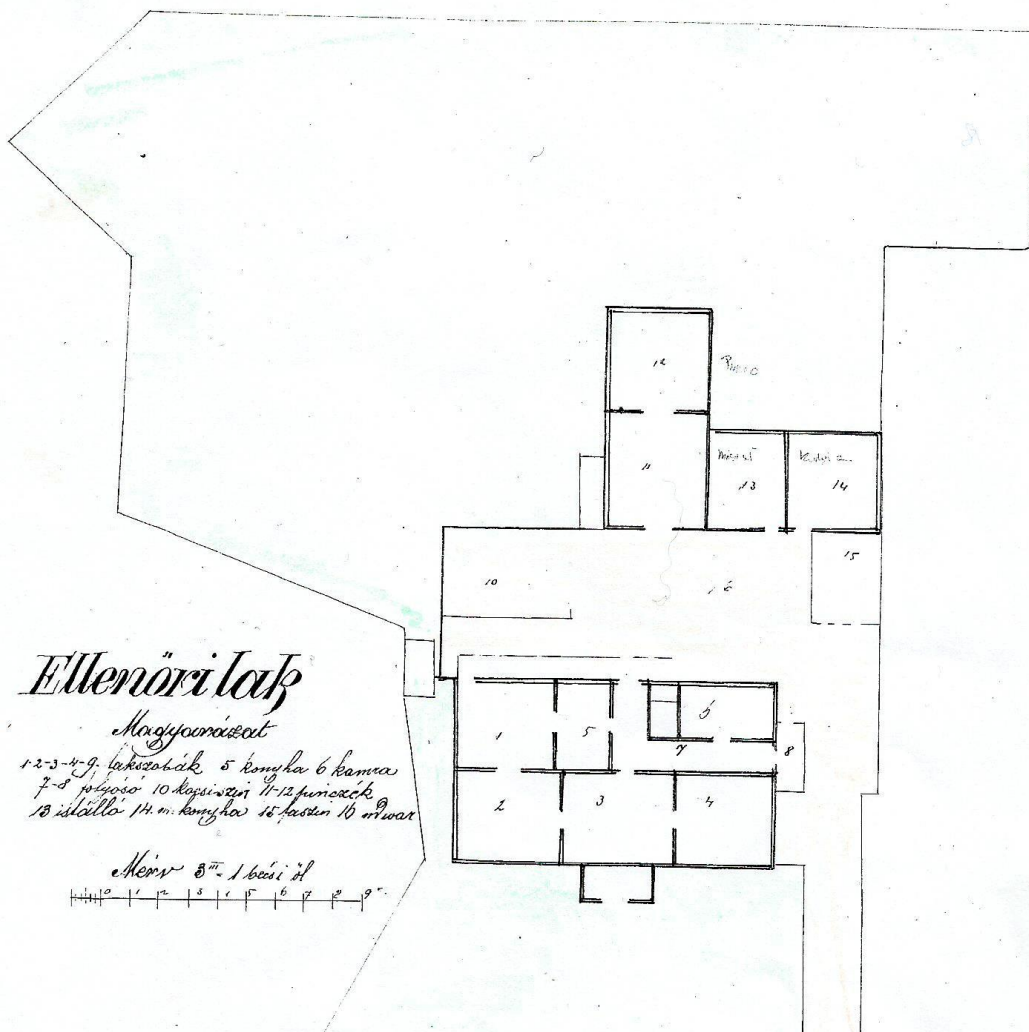
Obr. 37. Plán erárneho murovaného jednopodlažného domu v Tirolskej ulici nazývaný Kaštieľ určený pre honoráciu Hronca. Rozľahlý objekt s hospodárskym dvorom, s pivnicou, záhradou a predzáhradkou oddelenou od ulice vysokým múrom s oplotením. Strmá valbová strecha zastrešuje klenutý strop. Stavba naznačuje vek z prelomu 18. a 19. storočia.
