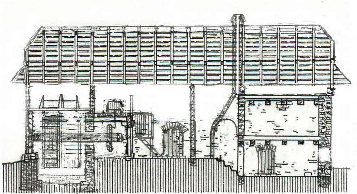
Obr. 20. Rez komorským mlynom v prednej časti (vpravo) od ulice s bytom mlynára v prízemí a skladovou sýpkou na poschodí. Vzadu (vľavo) kolesovňa a mlynica s dvomi kameňmi.
